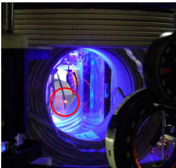
Figura 4. Encerclat amb un cercle vermell es pot veure la massa d'àtoms de rubidi atrapats per tres parells de feixos làser. És visible gràcies a la llum que emeten al ser excitats mitjançant els làsers. (Imatge: http://www.physics.utoronto.ca/~jhtgroup/labtour.html )
