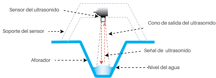
Figura 37. Funcionamiento de un sensor de ultrasonido.
