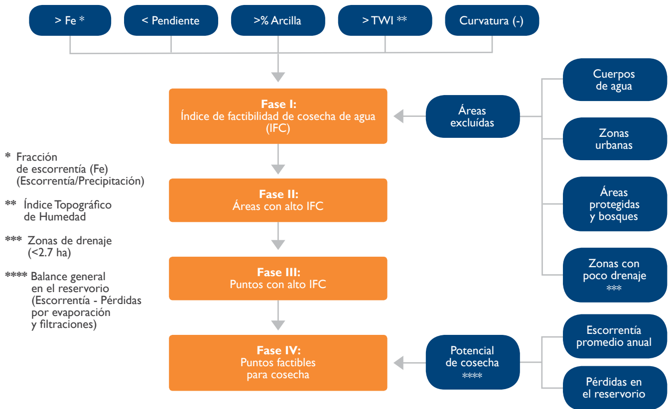
Figura I-3. Diagrama general para determinar sitios factibles para la cosecha de agua de escorrentía.
