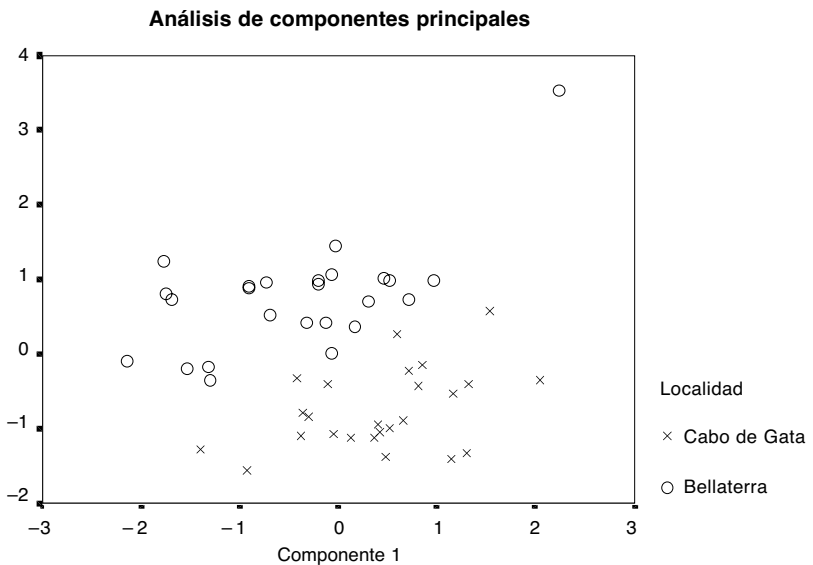
Figura 20. Distribución de los ejemplares en las dos primeras componentes.
