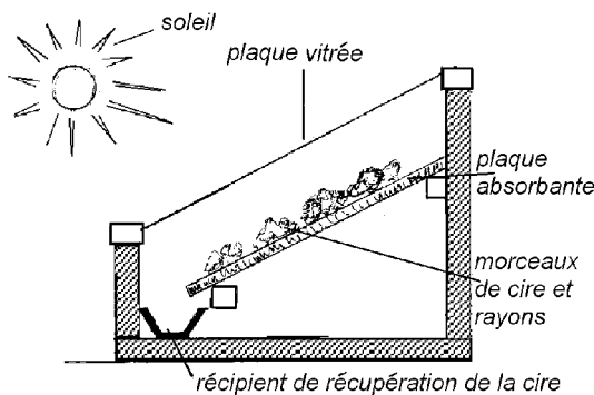
Figure 22 : Cérificateur solaire
