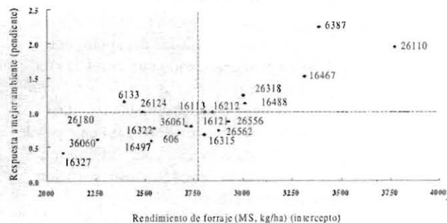
Figura 2. Clasificación de las accesiones de Brachiaria evaluadas durante la época de mínima precipitación en diferentes sitios de Colombia, basada en un Índice Ambiental (IA= pendiente de regresión lineal).
