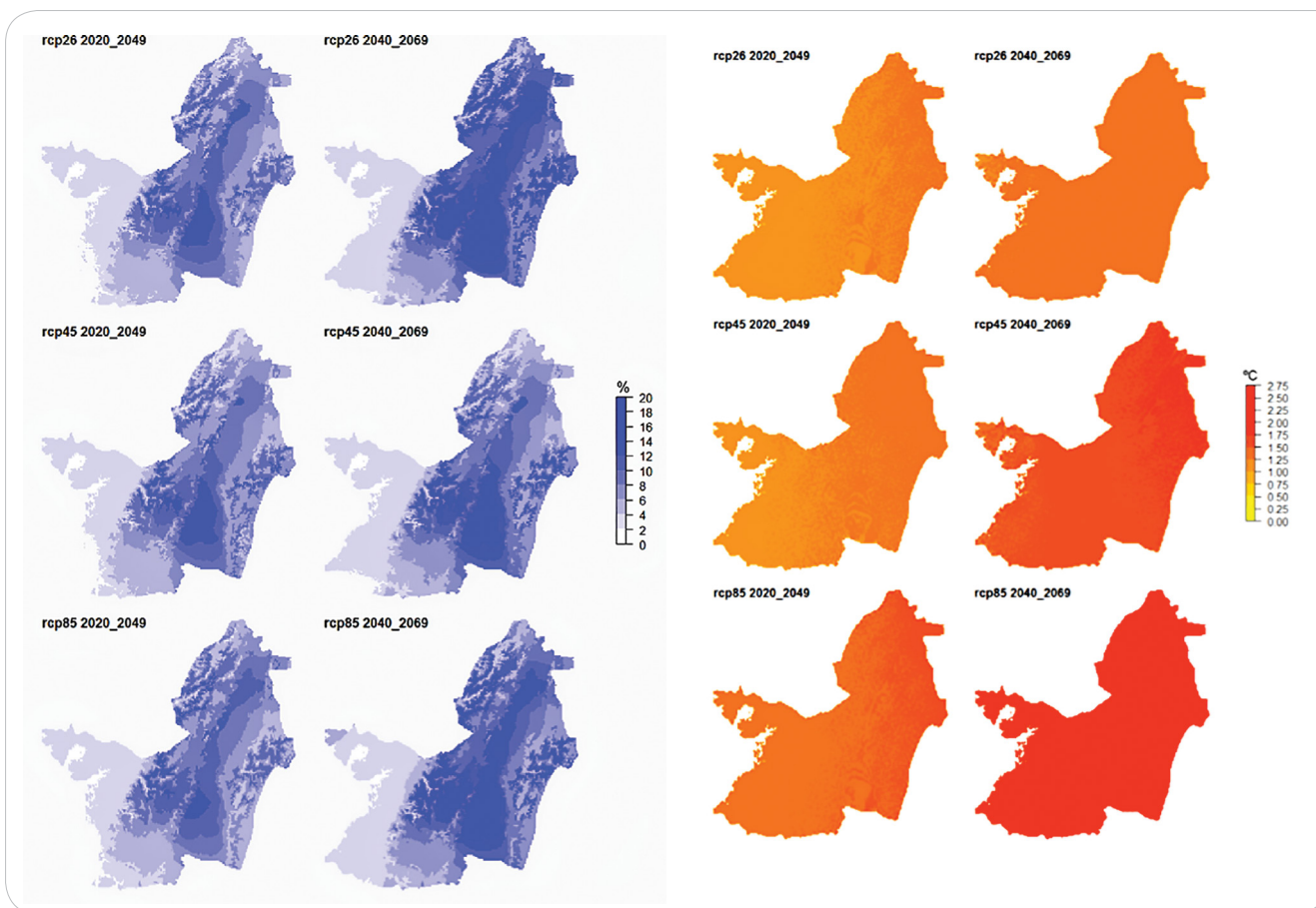
Figura 8. RCP 2.6, 4.5 y 8.5 para el Valle del Cauca. Años 2030 y 2050 (izquierda precipitación, derecha temperatura).
