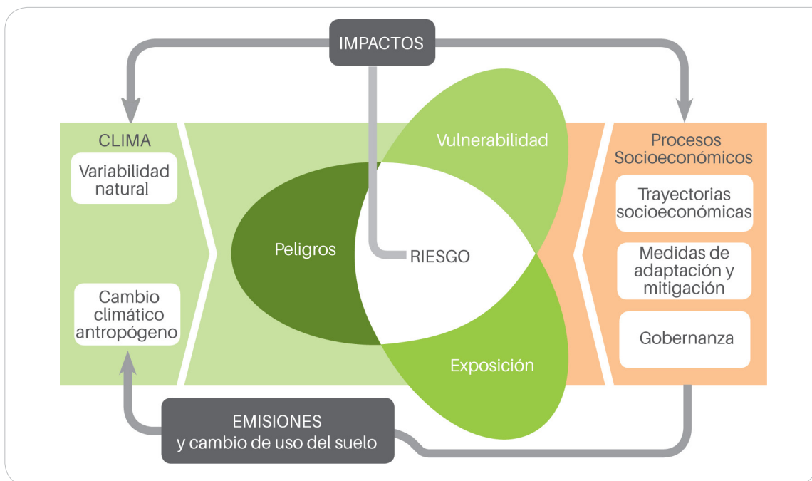
Figura 1. Esquema del análisis del riesgo a impactos de tipo climático, el cual se determina según la vulnerabilidad, los peligros y la exposición al fenómeno climático.
