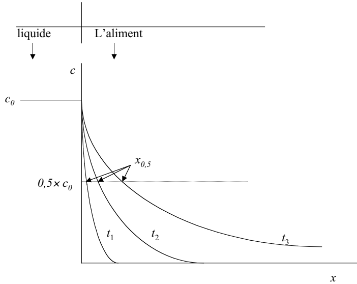
Figure 5.2.21 Changement de concentration c d'un composé migrant d'un liquide dans un aliment en fonction du temps ( t_1 < t_2 < t_3 ) et de la position x .
