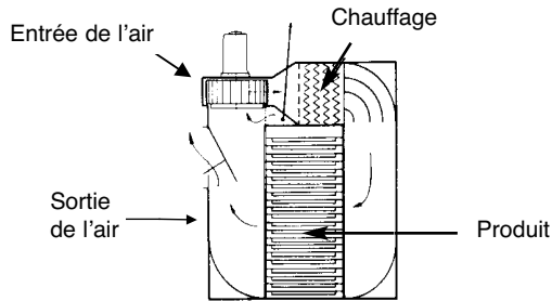
Figure 4.4.7 Étuve à sécher avec recirculation de l'air et chauffage électrique de l'air
