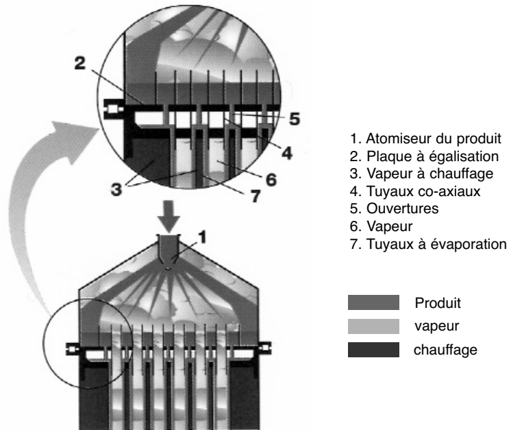
Figure 6.3 Section supérieure d'un évaporateur à couche mince à flux descendant
