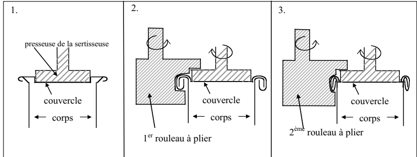
Figure 3.7.6 Le sertissage
