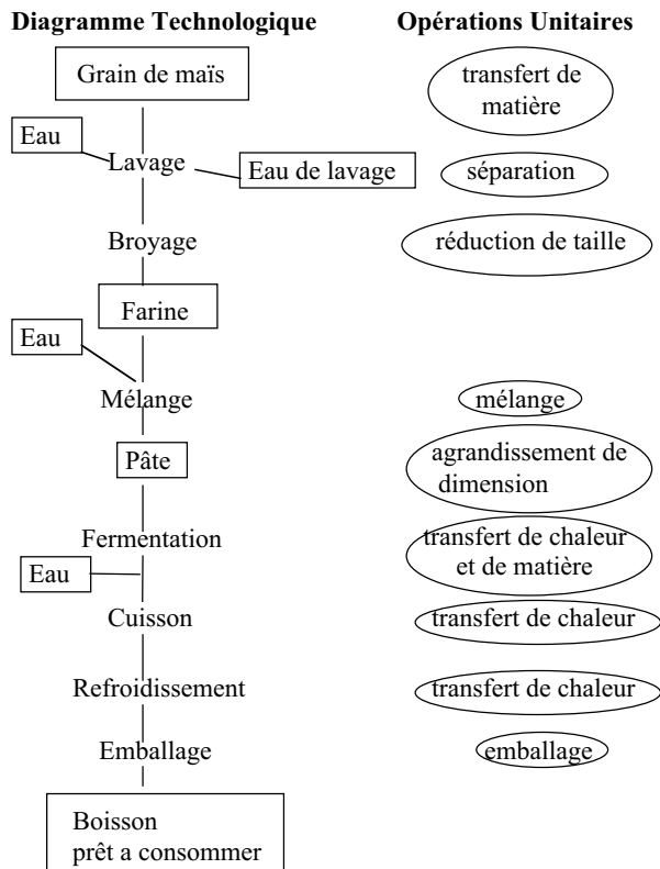
Figure 3.1.1 Diagramme technologique et Opérations Unitaires
