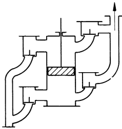
Figure 3.2.9 Pompe à piston
