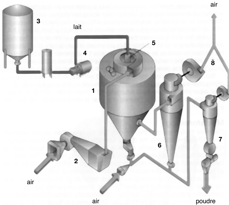
Figure 4.4.11 Séchoir à atomisation conventionnel
