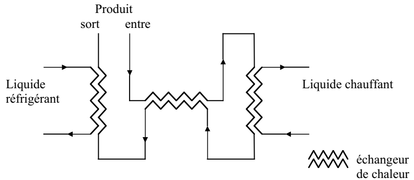
Figure 4.2.17 L'économie de la chaleur
