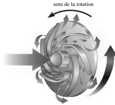
Figure 3.2.13 Principe du courant dans une pompe à force centrifuge
