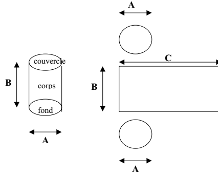
Figure 3.3.4 Calcul de superficie d'une boîte de conserve
