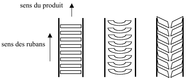
Figure 3.2.2 Profils des rubans (vue d'en haut)
