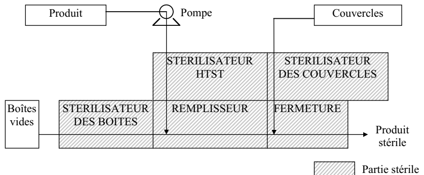
Figure 4.2.7 Mise en conserve stérile
