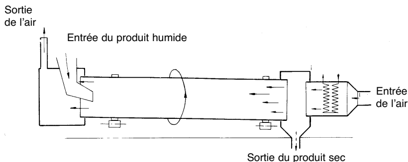
Figure 4.4.10 Séchoir à cylindre rotatoire
