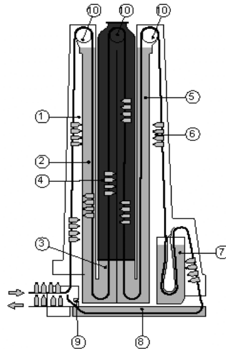
Figure 4.2.13 Stérilisateur vertical hydrostatique continu à bouteilles.
