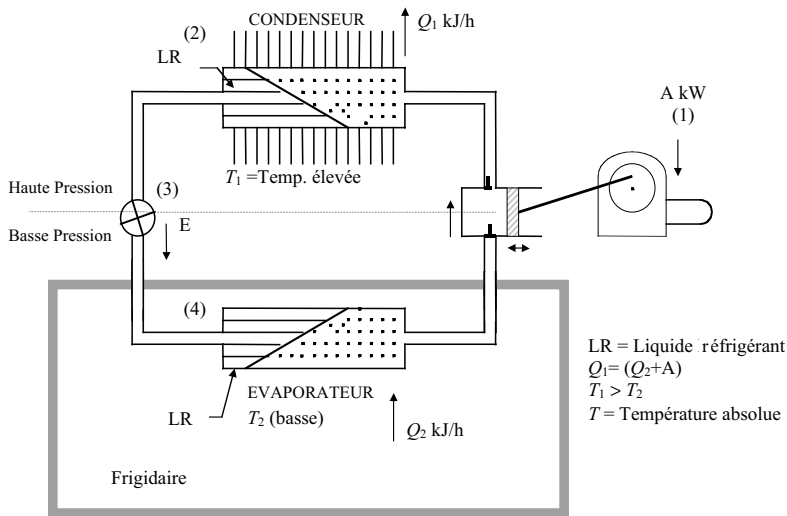
Figure 4.3.3 Système réfrigérant à compression
