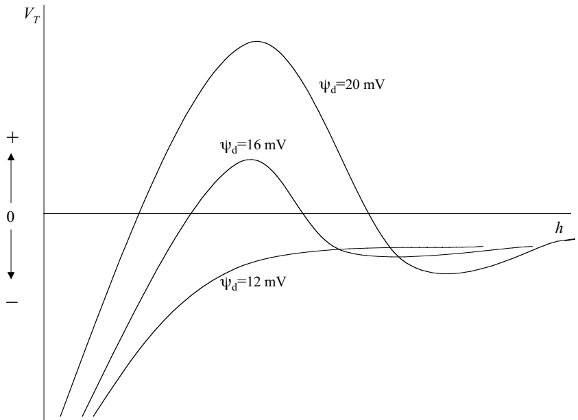
Figure 5.2.5 Exemple de l'effet de charge \psi_d sur l'énergie d'interaction V_T . Calculé pour deux globules avec r=2 \mu\text{m} et 1/\kappa=3 \text{ nm} (pas de répulsion stérique) mais les résultats sont seulement approximatifs.
