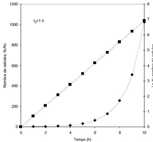
Figure 2.1.7 Déroulement linéaire et logarithmique de la phase exponentielle
