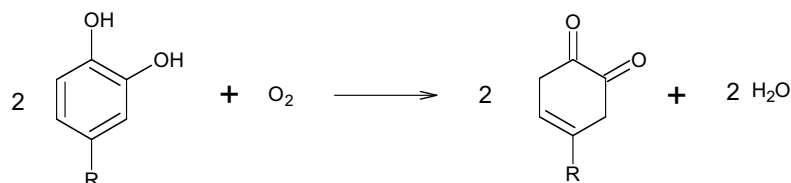
Fig. 2.3.17 L'étape d'oxydation dans le brunissement enzymatique
