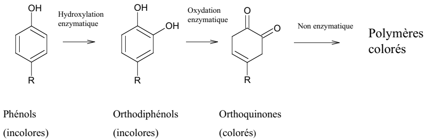
Fig. 2.3.16 Le brunissement enzymatique
