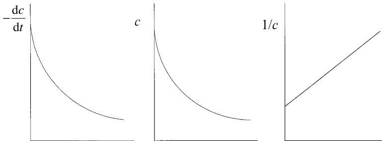
Figure 4.1.3 Une réaction d'ordre n=2
