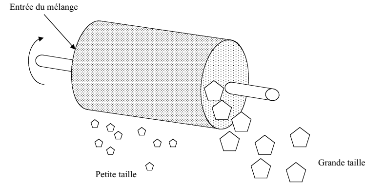
Figure 3.5.1 Tamis cylindrique
