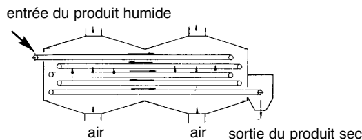
Figure 4.4.9 Séchoir à ruban
