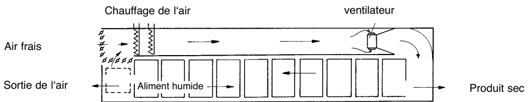
Figure 4.4.8 Séchoir à tunnel (Courants opposés)
