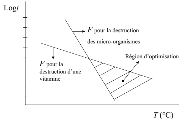
Figure 4.2.5 Diagramme représentant le problème d'optimisa- tion de traitement thermique
