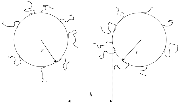
Figure 5.2.2 Figure représentant la répulsion dite stérique entre particules (très schématique et pas à l'échelle!)
