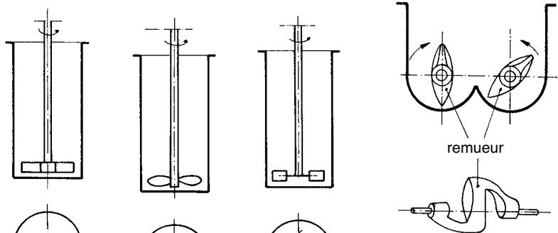
Figure 3.4.5 Agitateurs
