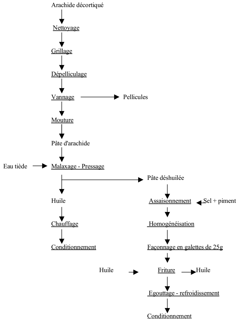
Figure 6.4.1 Diagramme de production d'huile d'arachide et de galettes « klui-klui »
