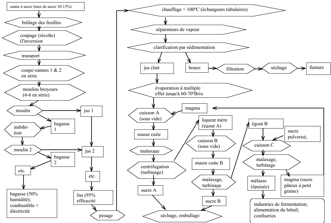
Figure 6.6.1 Diagramme technologique de la sucrerie
