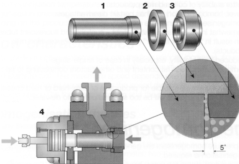
Figure 3.6.11 Les composants d'un homogénéisa- teur à action uni- que (1) Forceur, (2) Anneau de colli- sion (impacte), (3) Siège, (4) Presse hydro- lique
