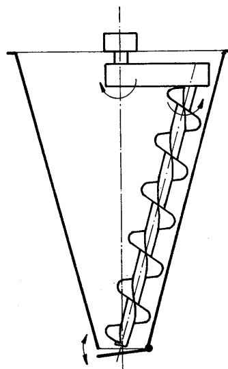
Figure 3.4.2 Mélangeur avec vis rotative
