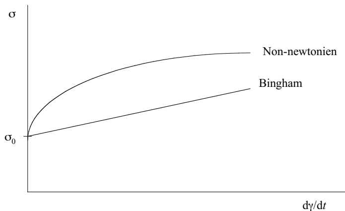
Figure 5.2.14 Représentation des corps plastiques
