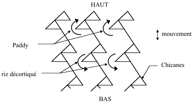
Figure 6.2.3 Table densimétrique vue d'en haut
