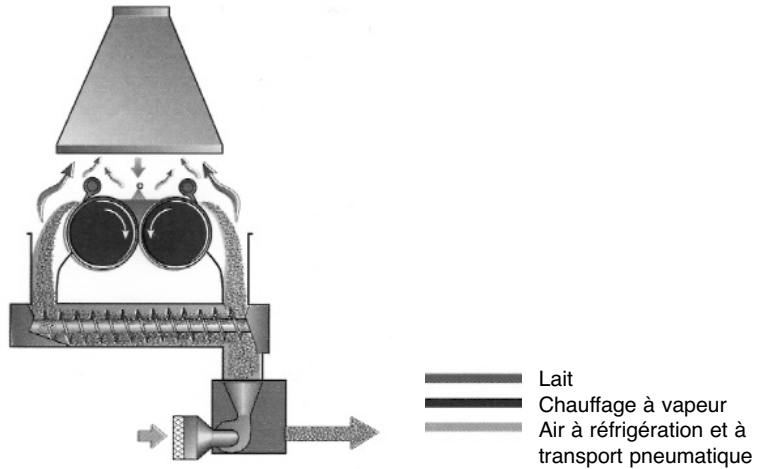
Figure 4.4.14 Principe d'un séchoir à double cylindre à alimentation continue
