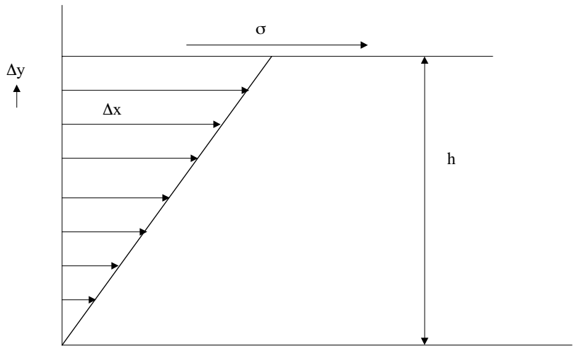
Figure 5.2.11 Représentation d'écoulement laminaire
