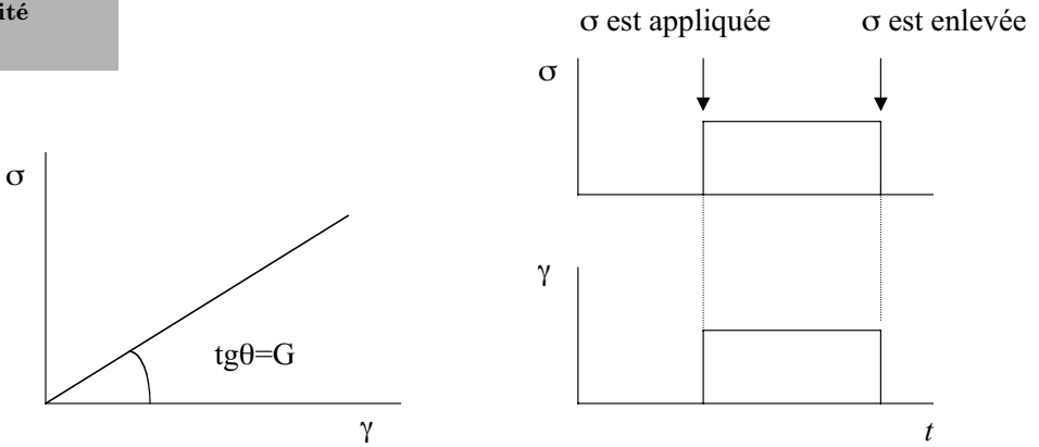
Figure 5.2.10 Représentation du comportement d'un solide élastique idéal
