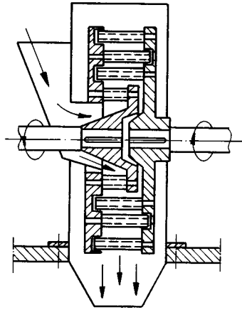
Figure 3.6.6 Désintégrateur
