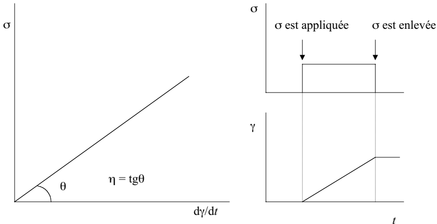
Figure 5.2.12 Représentation de la loi de Newton
