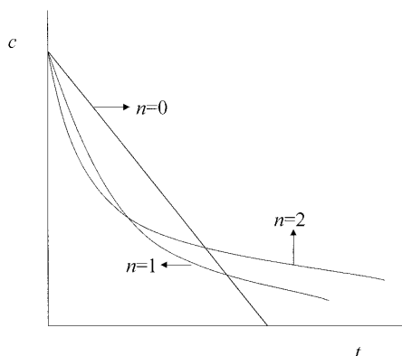
Figure 4.1.4 Comparaison des réactions d'ordre n=0,1 et 2
