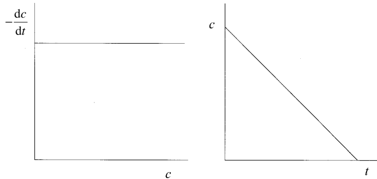
Figure 4.1.1 Une réaction d'ordre n=0
