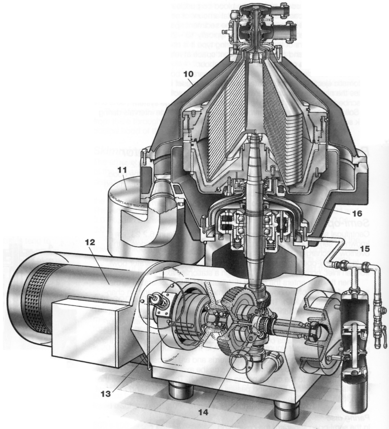
Figure 3.5.9 Centrifugeuse hermétique
