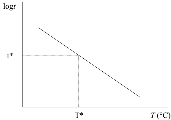
Figure 4.2.2 Diagramme selon le modèle de Bigelow
