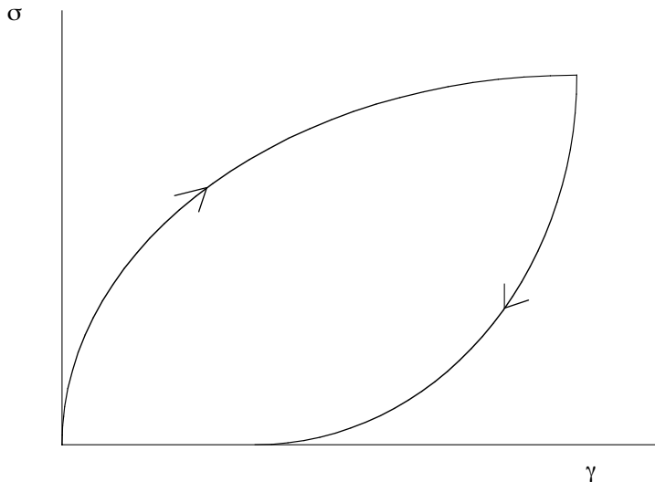
Figure 5.2.17 Représentation du comportement plastique
