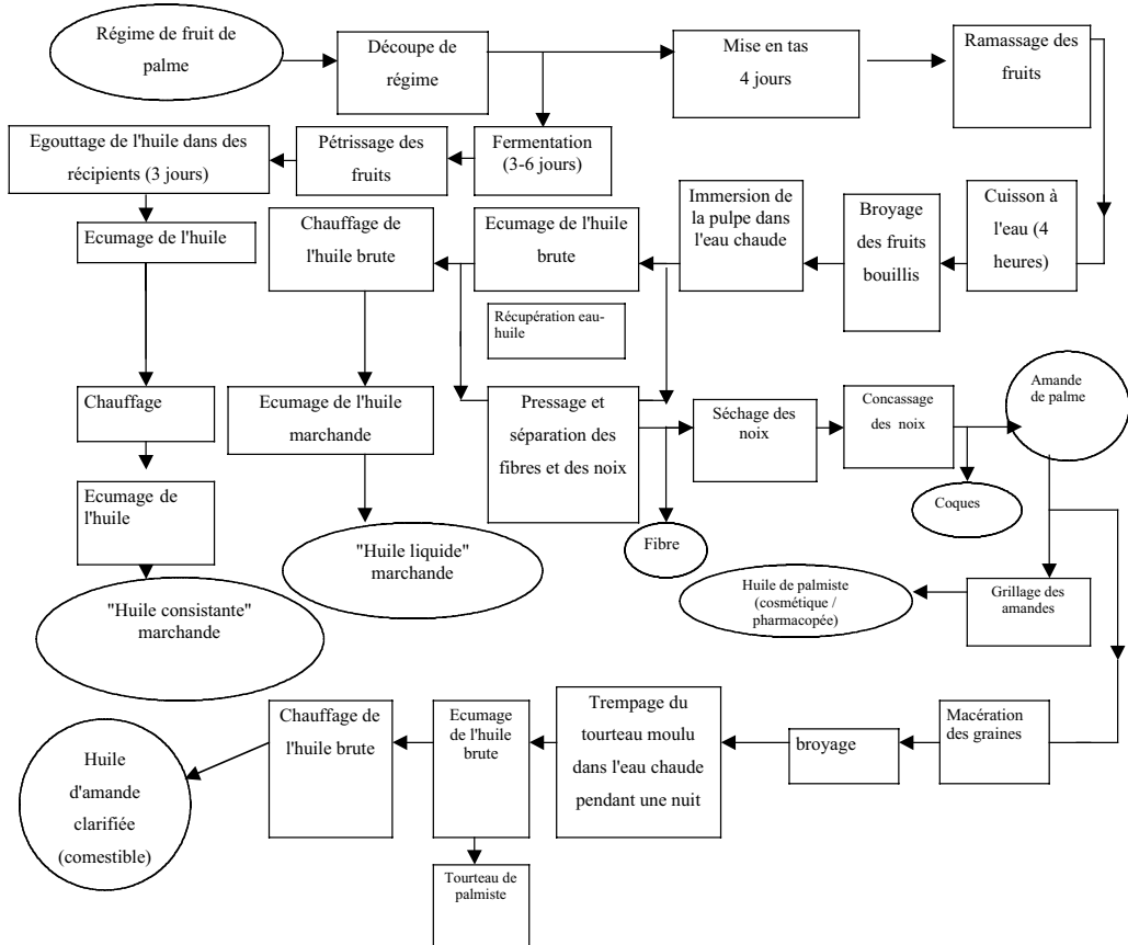
Figure 6.4.2 Schéma de traitement traditionnel des fruits de palmier
