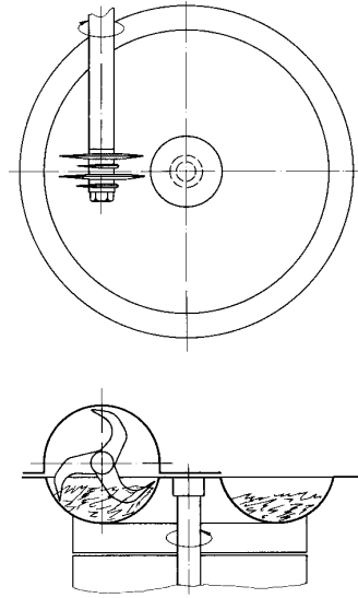
Figure 3.6.1 Coupeuse
