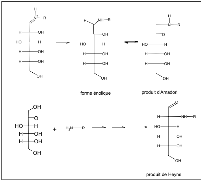
Figure 2.3.9 La réaction de Maillard (3). Le réarrangement d'Amadori (de Heyns)
