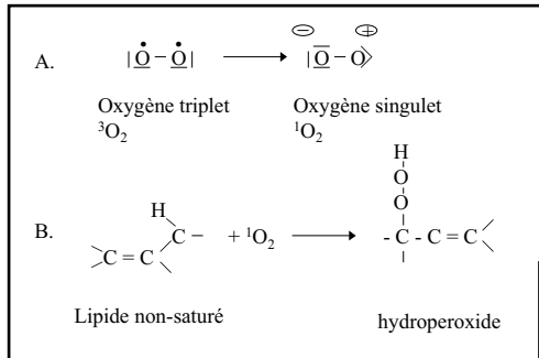
Fig. 2.3.1 Oxydation des lipides. A. Formation d'oxygène singulet B. Formation d'hydroperoxyde
