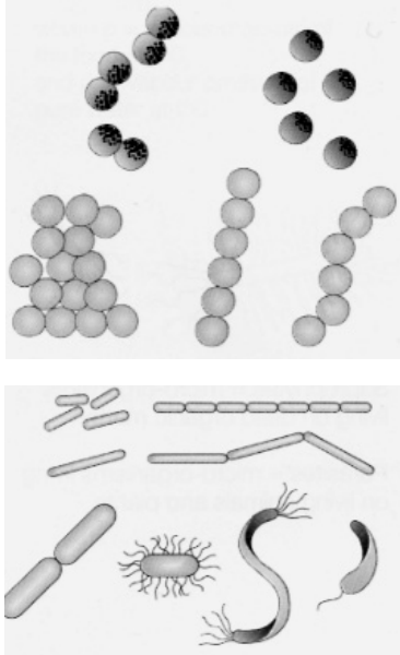
Figure 2.1.1 Les bactéries sphériques (coques) se présentent en divers groupements
