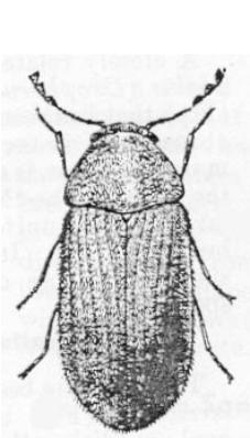
Fig. 2.4.10 Stegobium paniceum (adulte)
