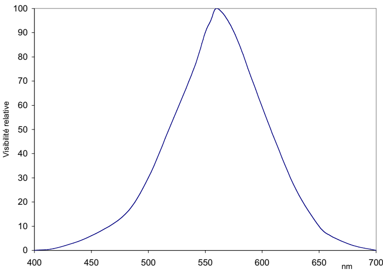
Figure 5.3.3 Courbe de la visibilité de l'œil humain
