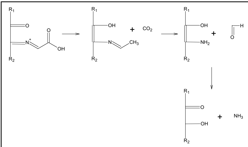
Figure 2.3.11 La réaction de Maillard (5). Dégradation de Strecker (suite)
