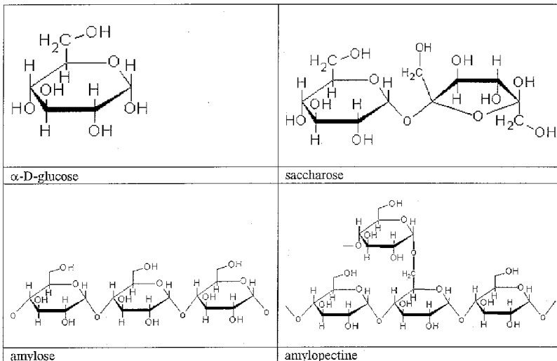
Figure 1.2.5 Structures de base de quelques saccharides
