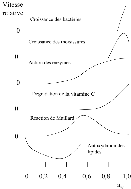
Figure 1.2.2 L'influence de l'activité de l'eau sur quelques réactions dans les aliments
