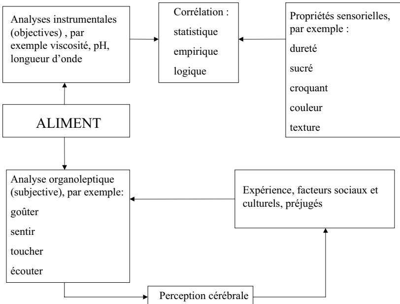
Figure 5.3.4 Schéma récapitulatif sur la mesure des propriétés organoleptiques.
