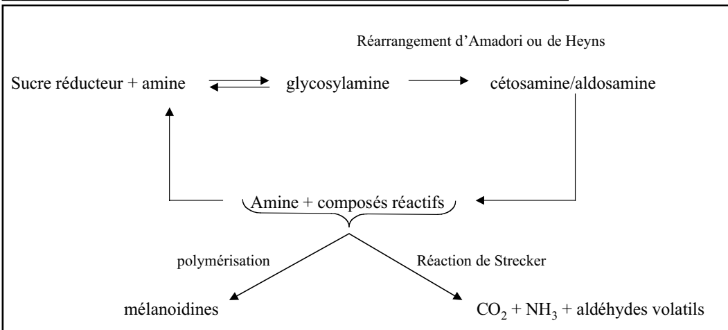
Figure 2.3.13 Résumé de la réaction de Maillard
