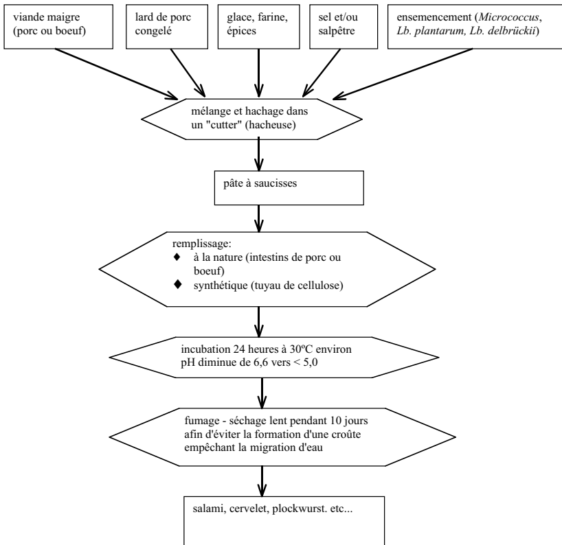
Figure 6.8.1 Diagramme de pro- duction de saucisses fermentées
