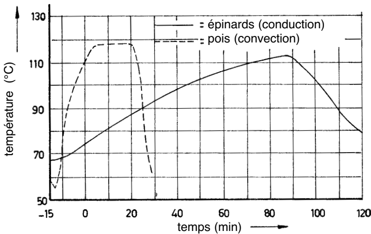
Figure 4.2.9 Températures à l'endroit le plus froid. Température autoclave 118°C, boîtes de 1 litre
