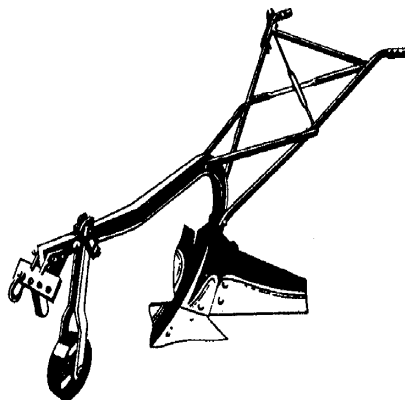
Figura 41: Sulcador “inkunki” de asa alta, fabricado no Zimbabue.
