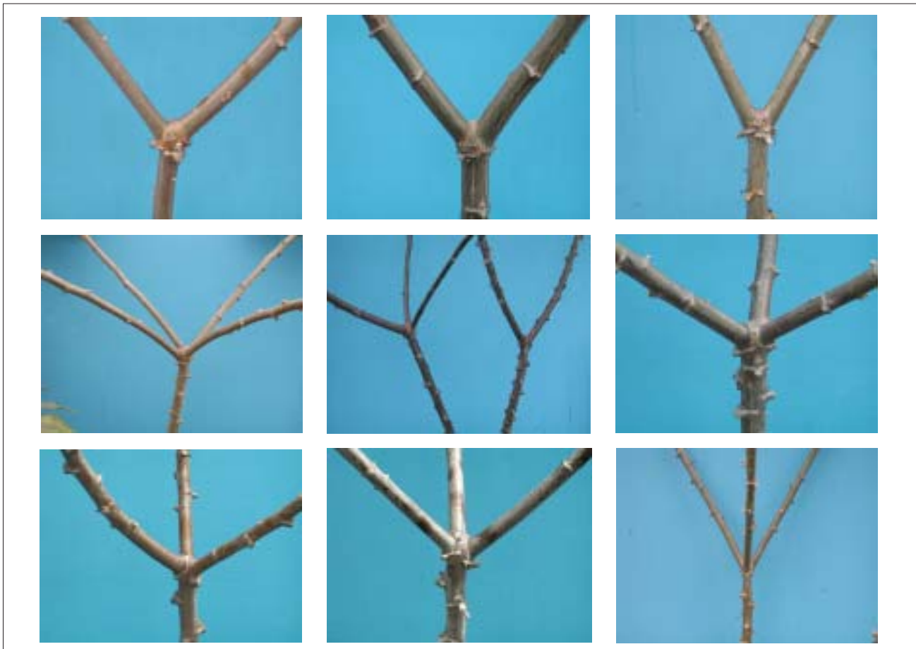
Figura 2-2. Variación en el número y ángulo de ramificación de la yuca.
