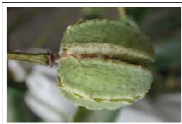
Figura 2-6. Fruto de la yuca.
