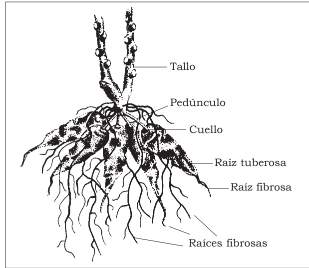
Figura 2-8. Componentes del sistema radical de la yuca.
