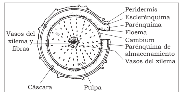
Figura 2-11. Corte transversal de una raíz tuberosa de yuca.
