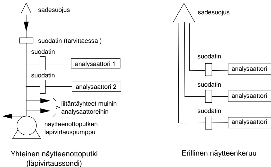
Kuva 3.2. Näytteenoton järjestäminen.
