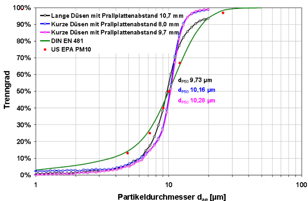
Kuva 3.1.a Hiukkasten leikkauskäyrä \text{PM}_{10} -mittauksissa erilaisilla inleteillä eli hiukkaskoon leikkureilla. Kuvan käyristä musta, sininen ja pinkki edustavat standardin EN 12341 mukaan valmistettuja inlettejä ja US EPA \text{PM}_{10} tarkoittaa Yhdysvalloissa hyväksytyä inlettä \text{PM}_{10} -mittauksille. Kuvaajan vaaka-akselilla on hiukkaskoko ja pystyakselilla läpäisyaste. (DIN EN 481 edustaa saksalaisen työilman hiukkaskoon määrittelyn mukaista inlettä).
