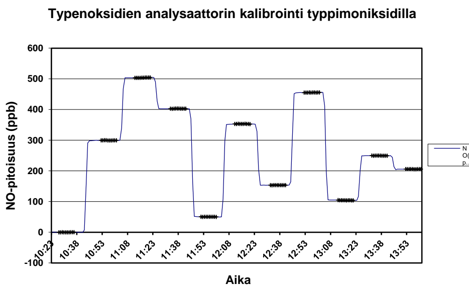
Kuva 4.2 Typen oksidien ( \text{NO} + \text{NO}_2 ) analysaattorin kalibrointi typpimonoksidilla. Kuvaan on merkitty analysaattorin mitaamat arvot minuuttiarvoina (jatkuva viiva) ja kalibrointipitoisuuksien laskemiseen tarvittavat pitoisuuskeskiarvot (++) kun pitoisuustaso on tasaantunut.
