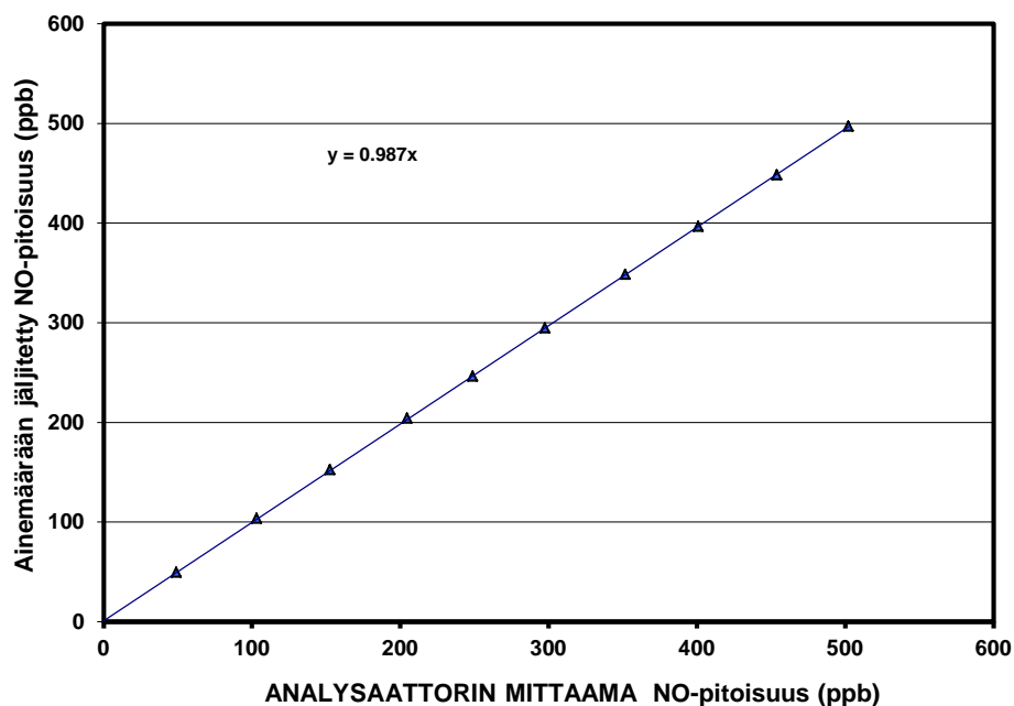
Kuva 4.3 Regressioanalyysin avulla laskettu analysaattorin mittaaman pitoisuuden ja kalibrointipitoisuuden välinen riippuvuus. Kun kalibrointipitoisuus sijoitetaan y-akselille ja analysaattorin mittaama pitoisuus x-akselille, kertoo regressiosuora suoraan, millä yhtälöllä analysaattorin tulokset on korjattava. Tämä on siis analysaattorin korjausyhtälö.
