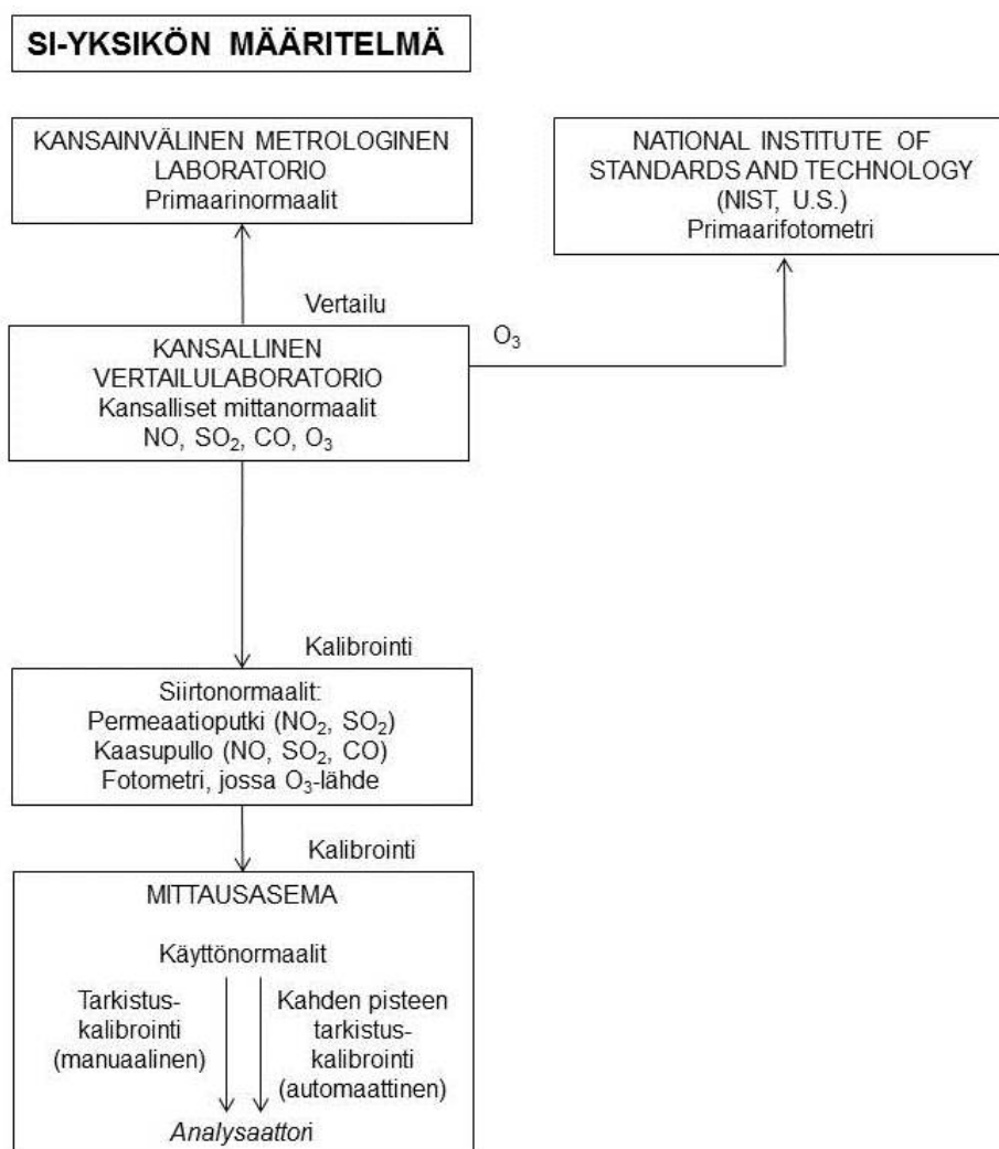
Kuva 4.1. Kaasunormaalien jäljitettävyyketju
