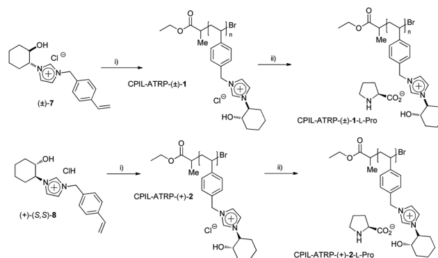
Scheme 2 ARGET-ATRP-polymerizations of CIL-monomers ((±)- 7 and (+)- S,S )- 8 ). (i) 60 °C, Et 2 PrBr, Cu 0 , CuBr 2 /tris(2-dimethylaminoethyl)amine (Me 6 TREN), [M] : [I] : [CuBr 2 ] : [L] 50 : 1 : 1 : 2. (ii) Amberlyst-OH, L -proline.
