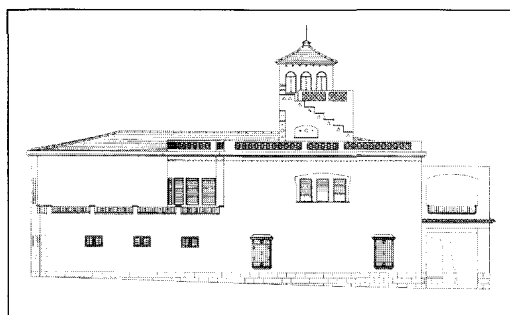
Figura 22 Alzado Oeste
