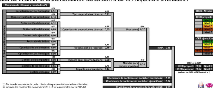
Fig. 1 Resultado de la evaluación de la sostenibilidad de la estructura del instituto de investigación
