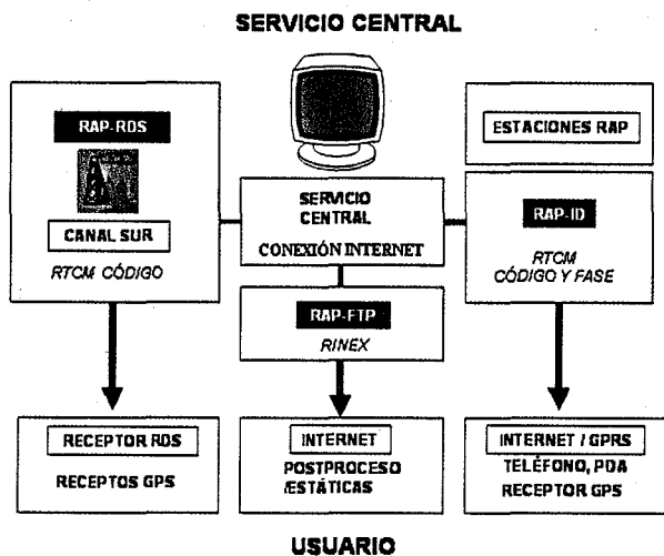
Componentes del centro de control de la RAP
