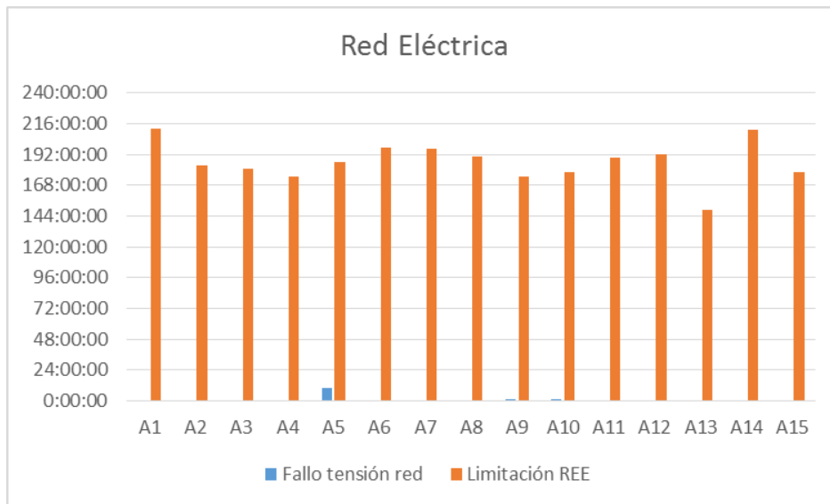
Gráfica 6. Horas parada Red Eléctrica por aerogenerador, Palomarejo
