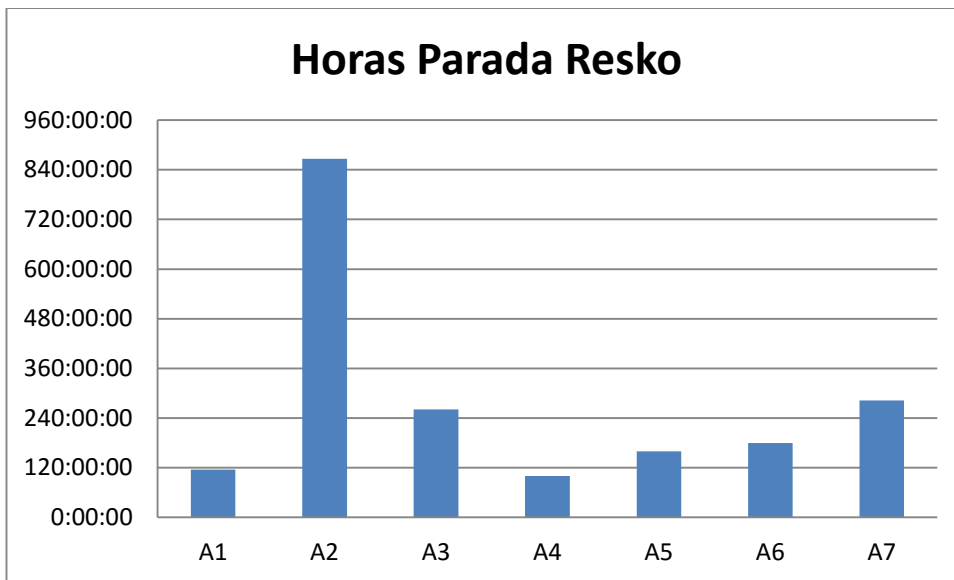
Gráfica 32. Horas parada total por aerogenerador Resko
