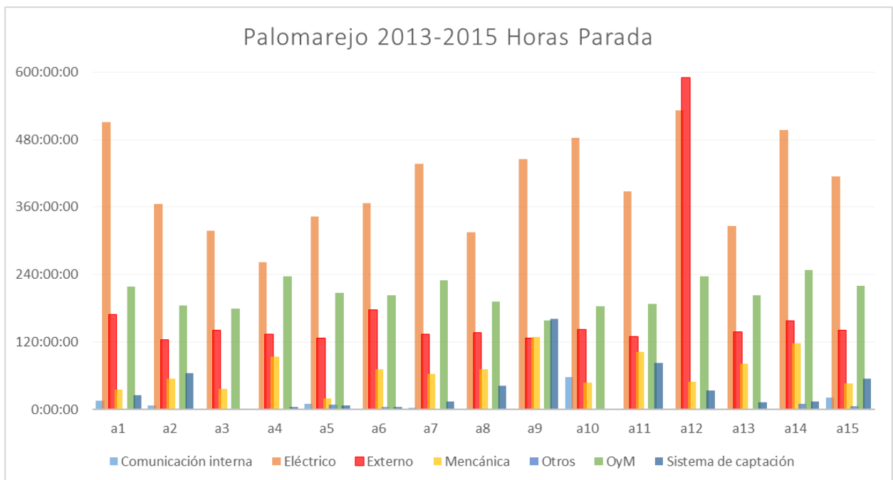
Gráfica 2. Horas de parada por aerogenerador y por sistema, Palomarejo
