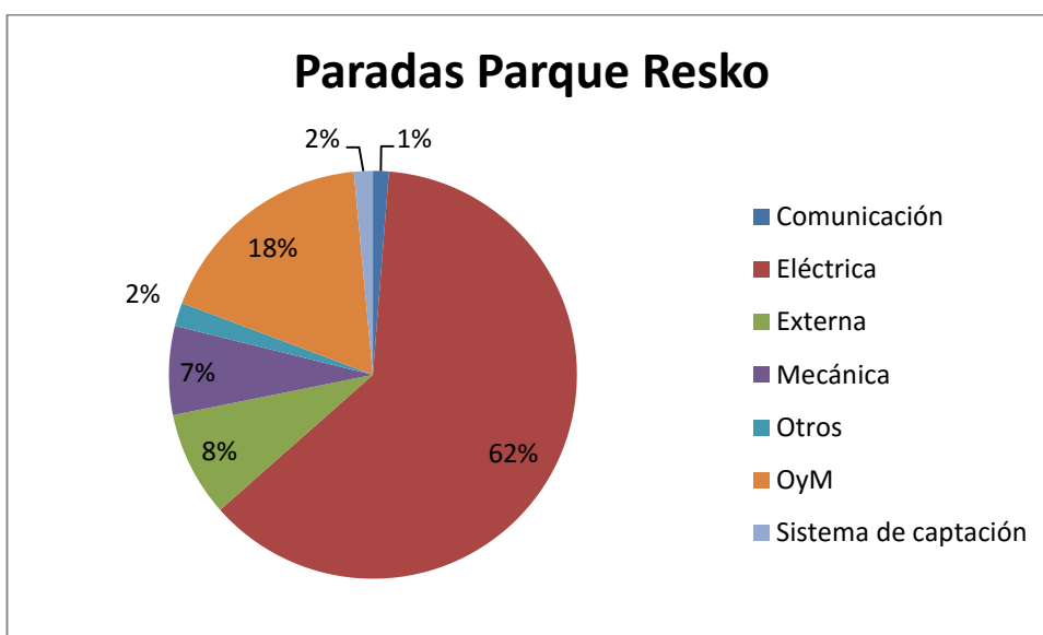
Gráfica 33. Porcentaje paradas por sistema Resko.
