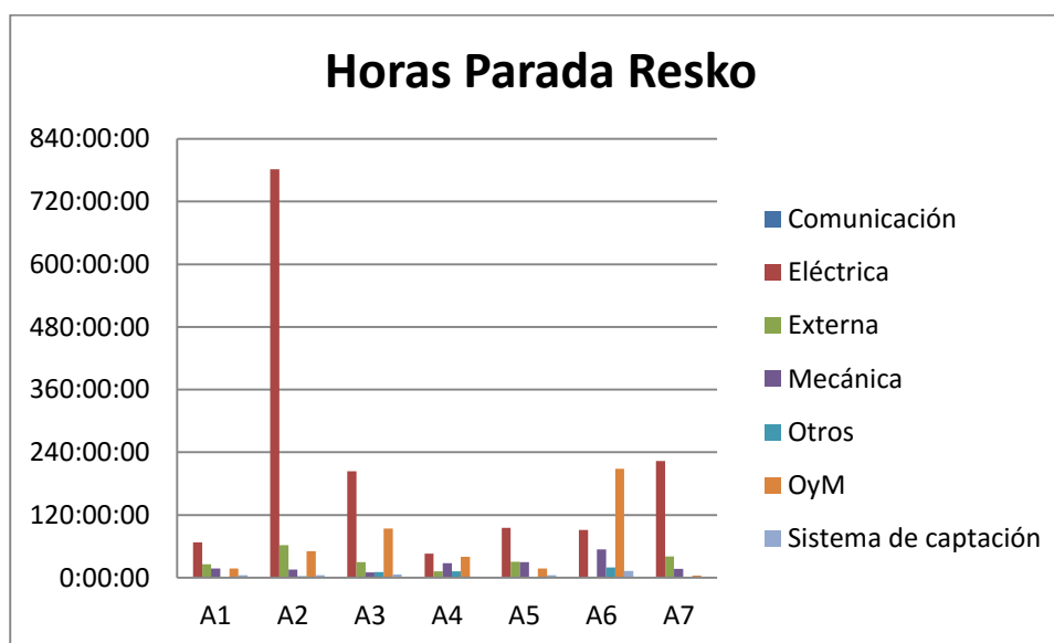
Gráfica 34. Horas parada por sistema por aero Resko.
