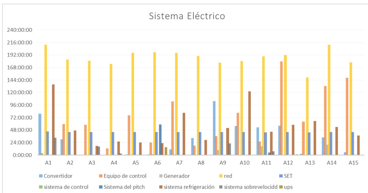
Gráfica 5. Horas Parada en el Sistema Eléctrico por aerogenerador, Palomarejo
