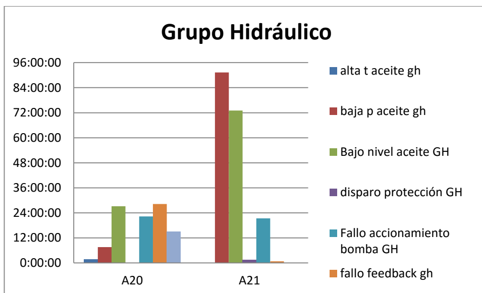
Gráfica 29. Horas parada Grupo Hidráulico A20 y A21, La Tella
