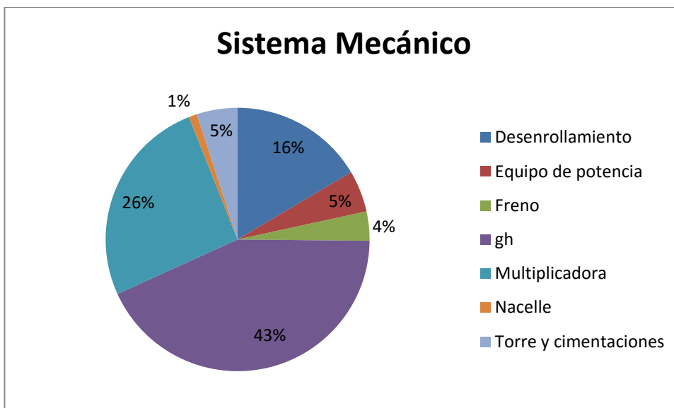
Gráfica 14. Porcentaje de paradas en el Sistema Mecánico, Palomarejo
