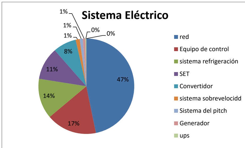
Gráfica 4. Porcentaje paradas en el Sistema Eléctrico, Palomarejo
