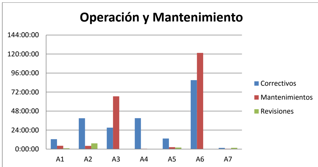
Gráfica 37. Horas parada Operación y Mantenimiento Resko
