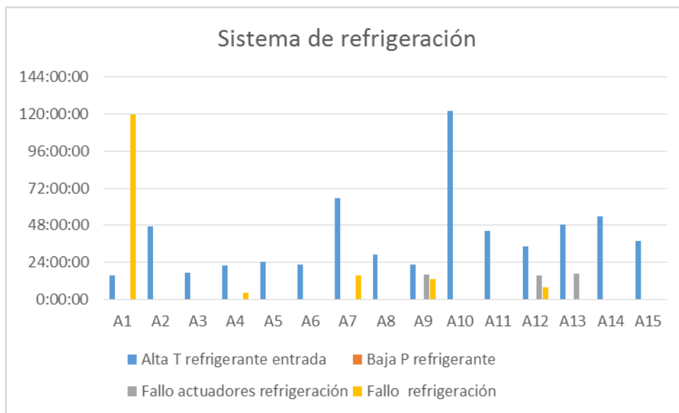
Gráfica 10. Horas de parada en el Sistema de Refrigeración por aerogenerador, Palomarejo
