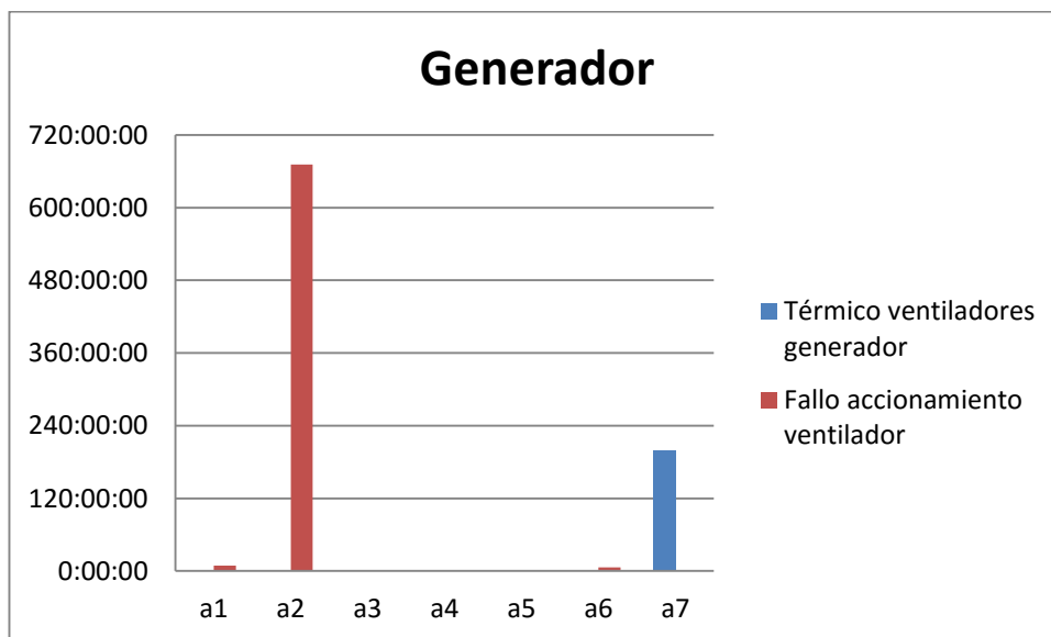
Gráfica 36. Horas parada Generador por aerogenerador Resko
