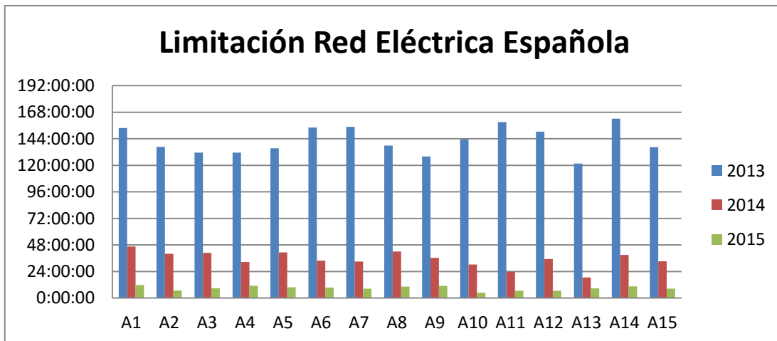
Gráfica 7. Horas parada Limitación REE por aerogenerador por año, Palomarejo
