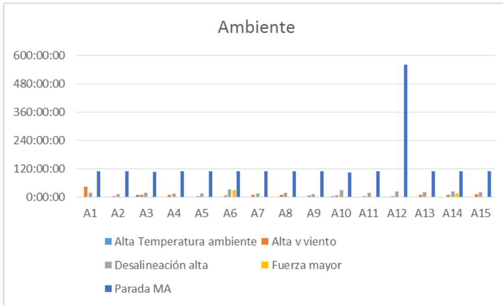
Gráfica 13. Horas de parada debido a problemas Ambientales por aerogenerador, Palomarejo
