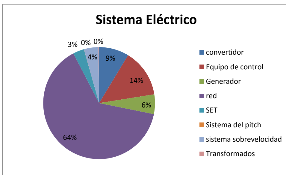
Gráfica 21. Porcentaje de paradas en el Sistema Eléctrico, La Tella
