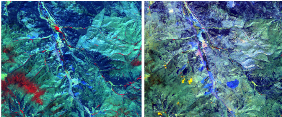
Рис.1. Комбинации каналов снимков Landsat 4-5, Landsat 8 для выявления наледей. Слева – наледи на реке Брянке в 1998 году, справа – тот же участок в 2013 г.
