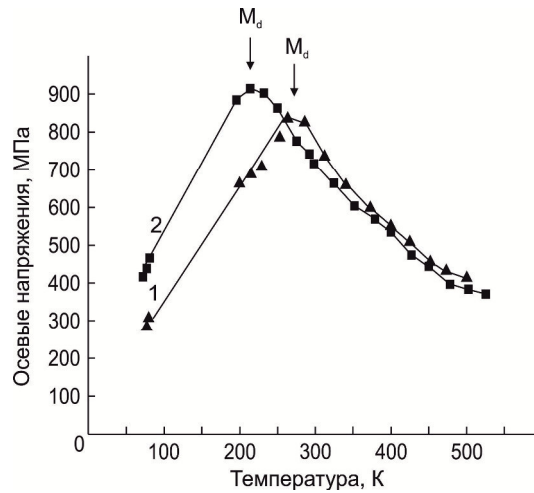
Рис.1 Температурная зависимость осевых напряжений \sigma_{0,1}(T) для [001]-ориентации монокристаллов сплава: 1 – Ta , 2 – TaV, состаренных при T=973 К в течение 30 минут при деформации растяжением
