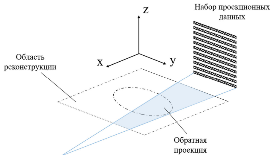
Рис. 3. Обратное проецирование данных, полученных на коллированном пучке
