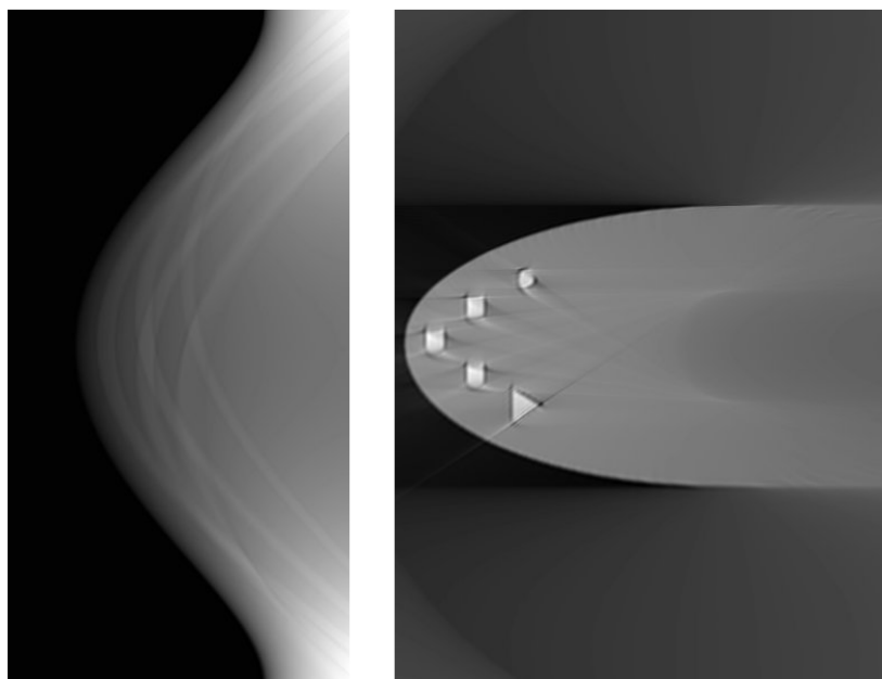
Рис. 4. Слева – синограмма, полученная на коллимированном пучке, справа – реконструкция отсканированной части объекта
