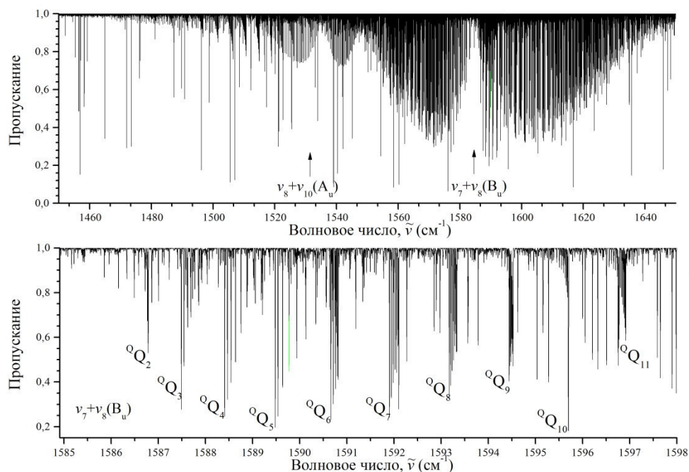
Рис. 1. Активные в инфракрасном поглощении колебательно-вращательные полосы молекулы транс- C_2H_2D_2 в области 1450-1650\text{ см}^{-1} .
