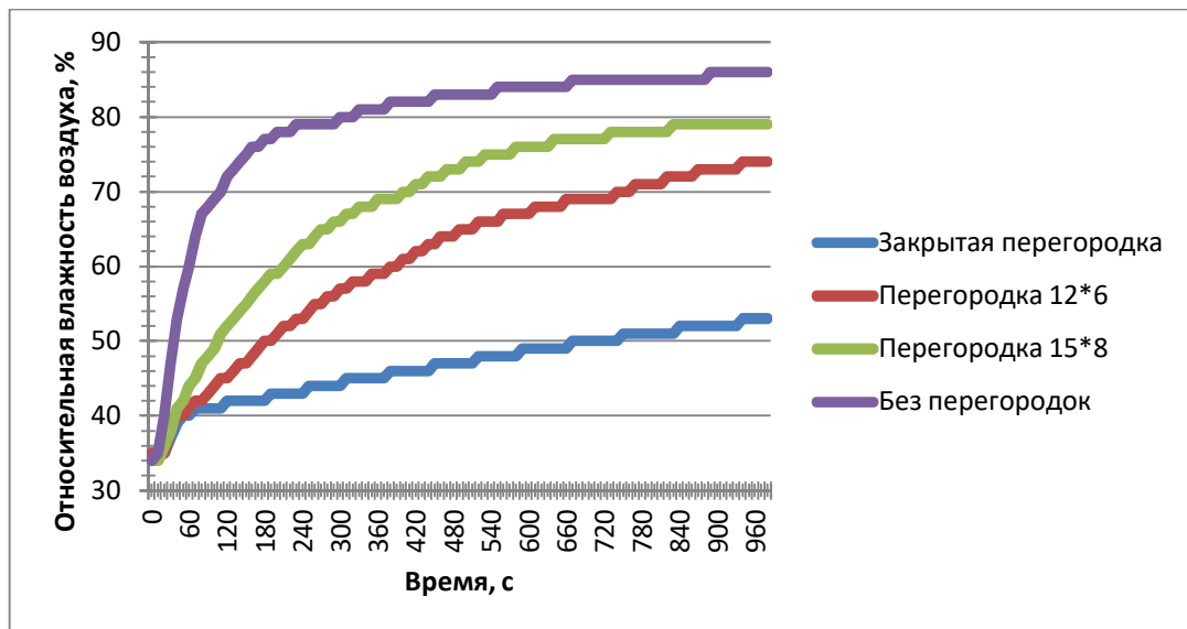
Рисунок 9 – Зависимость относительной влажности воздуха от времени, при различной площади открытой поверхности перегородок
