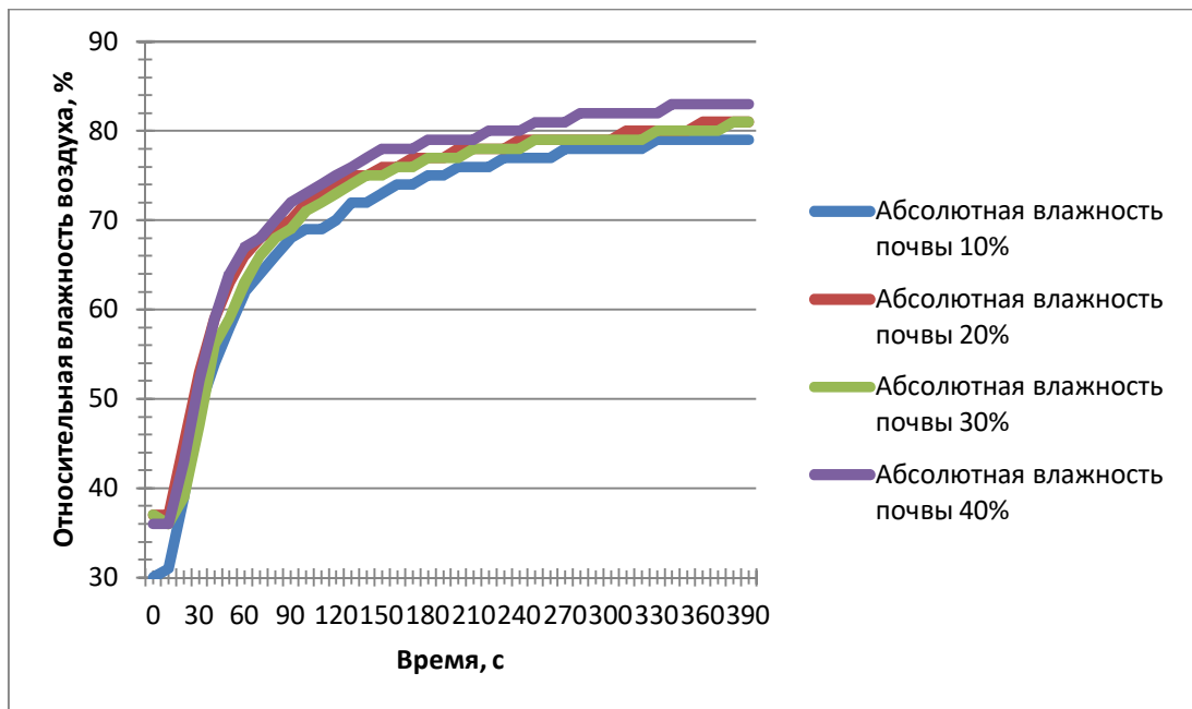
Рисунок 7 – Зависимость относительной влажности воздуха от времени
