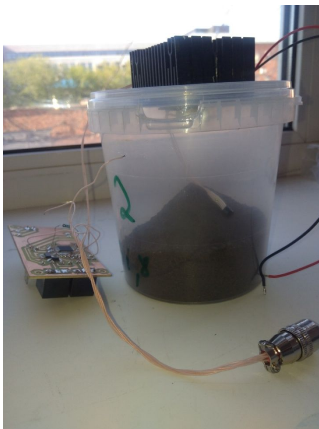
Рисунок 12 – Измерение влажности почвы методом точки росы в закрытой системе
