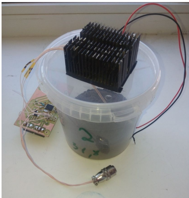
Рисунок 11 – Измерение влажности почвы методом точки росы в закрытой системе
