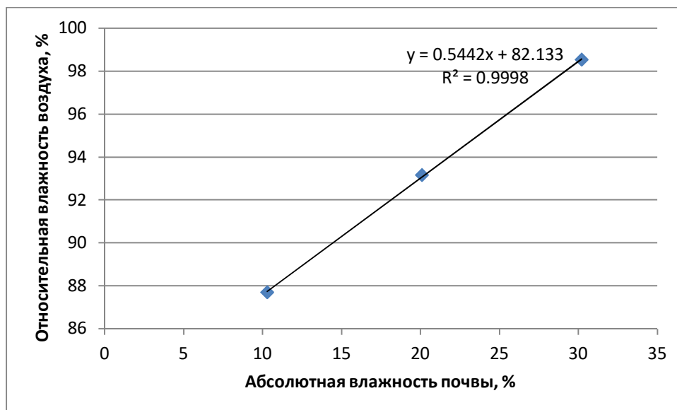
Рисунок 13 – Зависимость относительной влажности воздуха от абсолютной влажности суглинистой почвы
