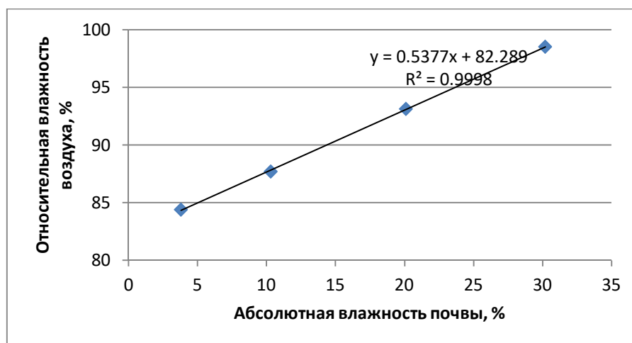
Рисунок 14 – Зависимость относительной влажности воздуха от абсолютной влажности песка, суглинистой почвы и чернозема
