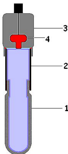
Рисунок 1 – Схема устройства тензиометра
