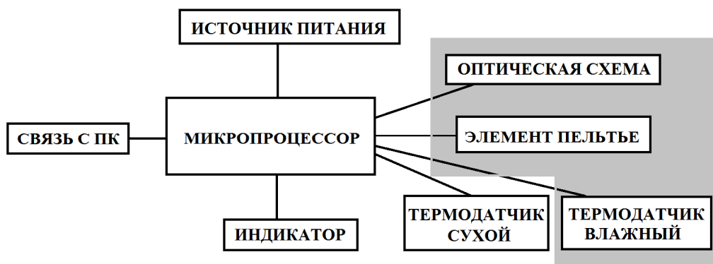
Рисунок 2 – Схема измерителя влажности почвы по методу точки росы
