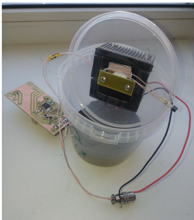
Рисунок 10 – Прибор измерения влажности воздуха методом точки росы
