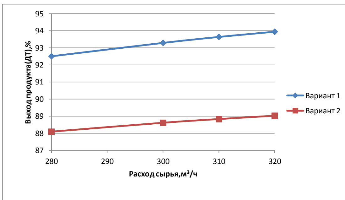
Рисунок 3.6 – Зависимость выхода продукта (ДТ) от расхода сырья
