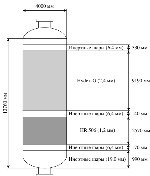
Рисунок 2.2 – Схема реактора каталитической депарафинизации
