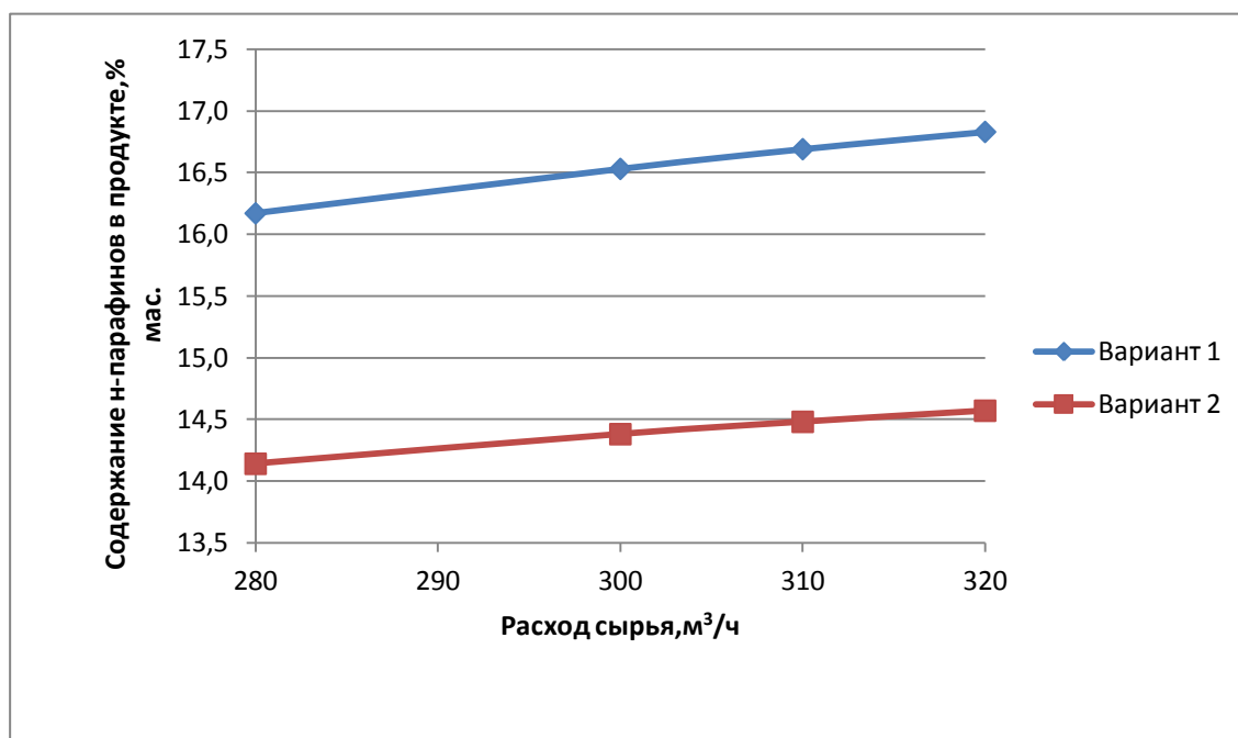
Рисунок 3.4 – Зависимость содержания н-парафинов в продукте от расхода сырья
