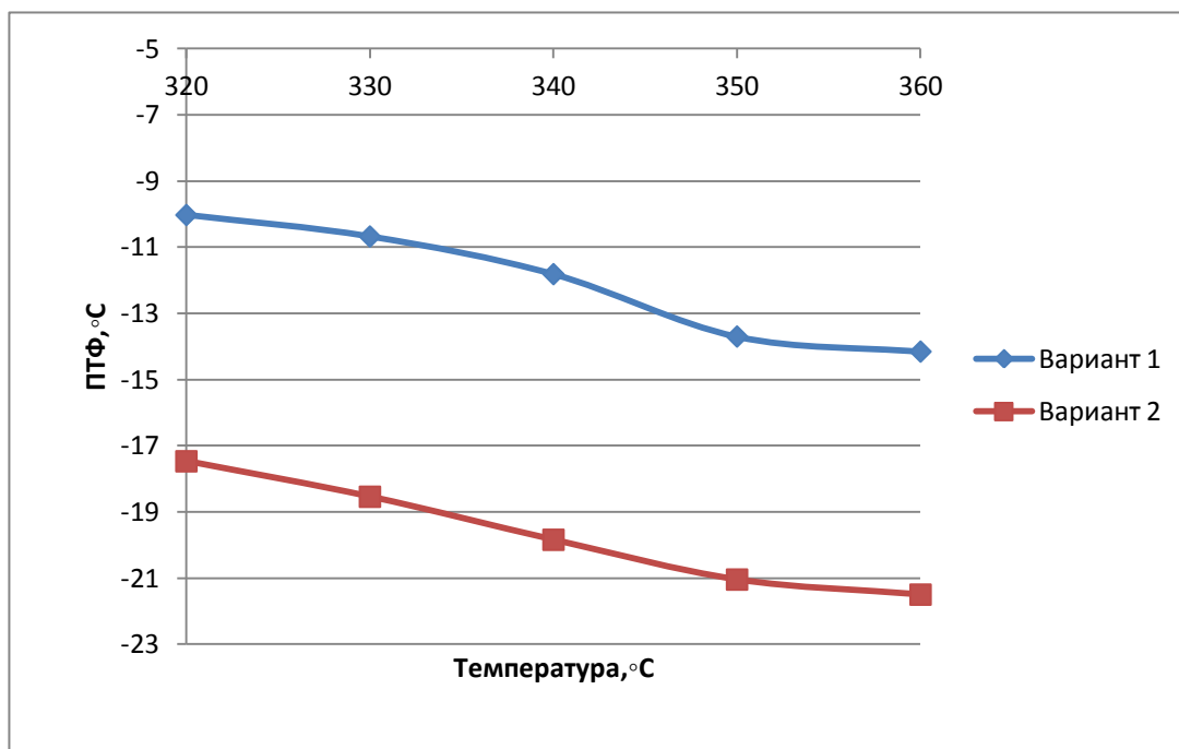
Рисунок 3.2 - Зависимость ПТФ от температуры процесса
