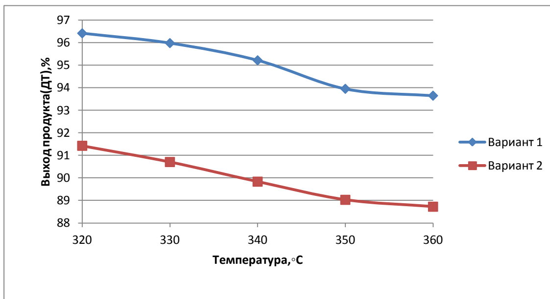
Рисунок 3.3– Зависимость выхода продукта (ДТ) от температуры процесса
