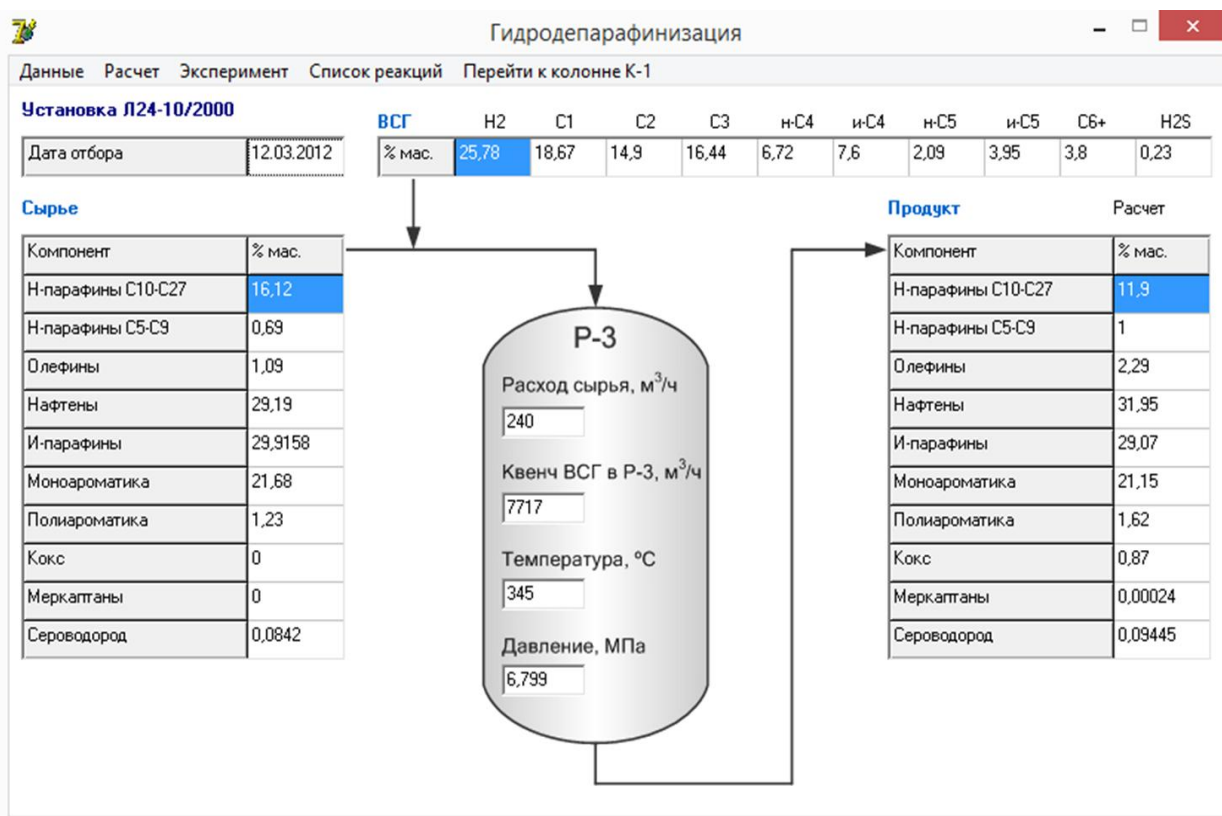
Рисунок 2.3 - Интерфейс компьютерной моделирующей системы процесса гидродепарафинизации
