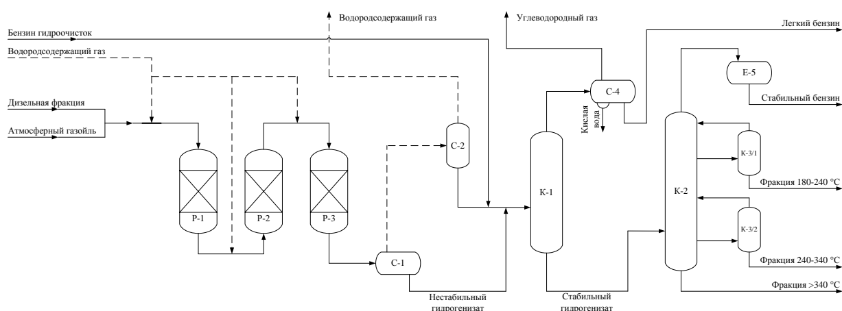
Рисунок 2.1 – Схема основных потоков установки каталитической депарафинизации ООО «ПО «Киришинефтеоргсинтез»
