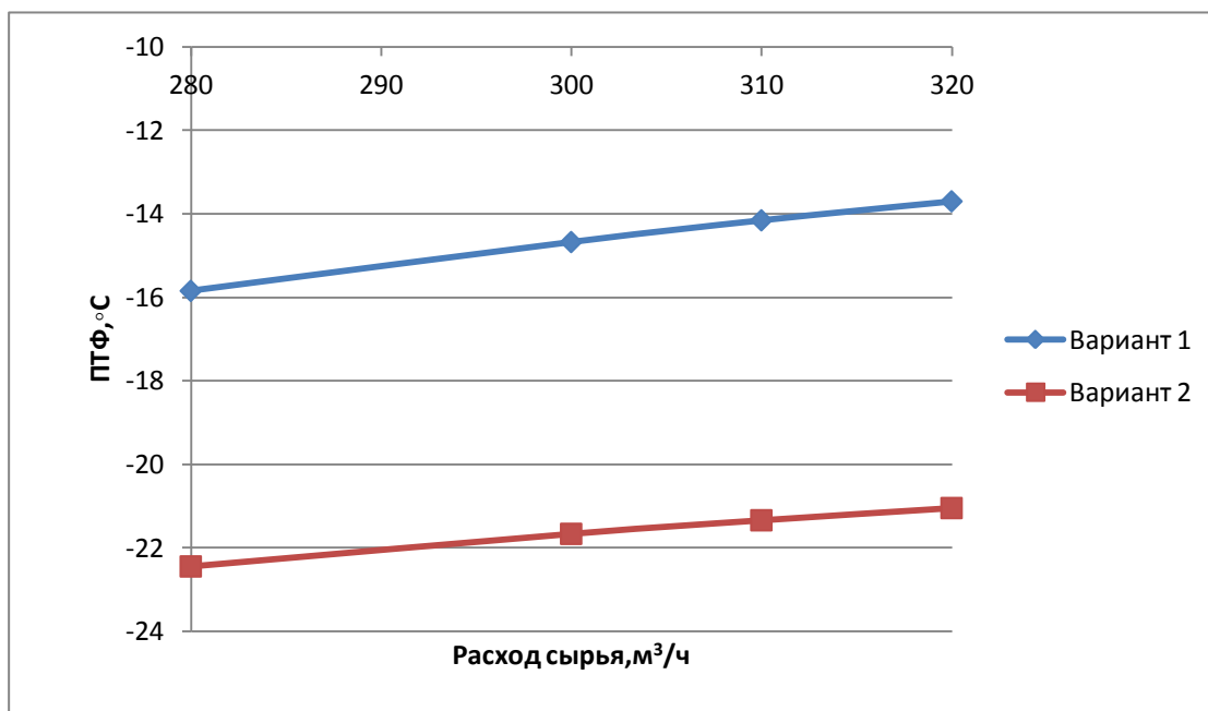
Рисунок 3.5 – Зависимость ПТФ продукта от расхода сырья
