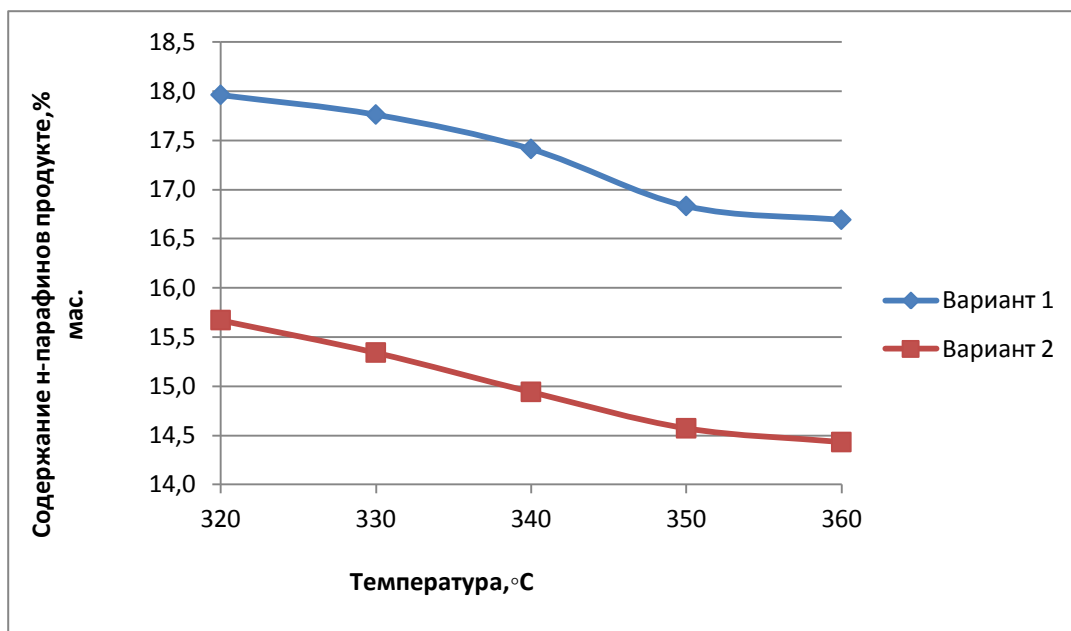
Рисунок 3.1 - Зависимость содержания н-парафинов от температуры процесса
