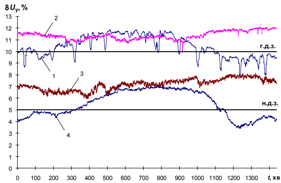
Рис. 1. Усталене відхилення напруги на шинах 110 кВ чотирьох різних підстанцій
