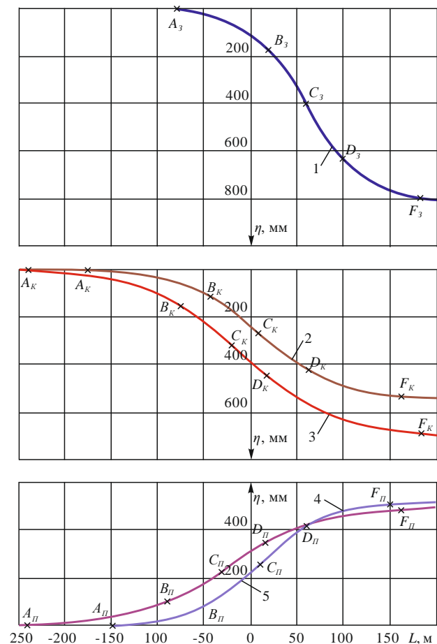
Рисунок 3. Зависимости оседания точек земной поверхности и сдвижения пород на контуре подготовительных выработок ( \eta ) от их положения относительно очистного забоя ( L ) в условиях шахты “Степная”: 1 – кривая оседания земной поверхности; 2, 4 – кривые сдвижения кровли и почвы на контуре 159-го штрека; 3, 5 – кривые сдвижения кровли и почвы на контуре 163-го штрека; A_n, B_n, C_n, D_n, F_n – характерные точки сдвижения пород почвы; A_k, B_k, C_k, D_k, F_k – характерные точки сдвижения пород кровли; A_3, B_3, C_3, D_3, F_3 – характерные точки оседания земной поверхности
