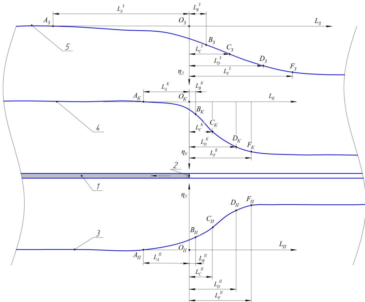
Рисунок 1. Схема оседания земной поверхности и сдвигения пород кровли и почвы участковой выработки относительно очистного забоя: 1 – разрабатываемый пласт; 2 – очистной забой; 3, 4, 5 – кривые, характеризующие соответственно сдвигение почвы и кровли участковой выработки, и оседание земной поверхности; L_{II} , L_K , L_3 – оси абсцисс соответственно для почвы и кровли выработки, и земной поверхности; \eta_{II} , \eta_K , \eta_3 – оси ординат соответственно для почвы и кровли выработки, и земной поверхности; A_{II} , B_{II} , C_{II} , D_{II} , F_{II} – характерные точки кривой сдвигения почвы; A_K , B_K , C_K , D_K , F_K – характерные точки кривой сдвигения кровли; A_3 , B_3 , C_3 , D_3 , F_3 – характерные точки оседания земной поверхности
