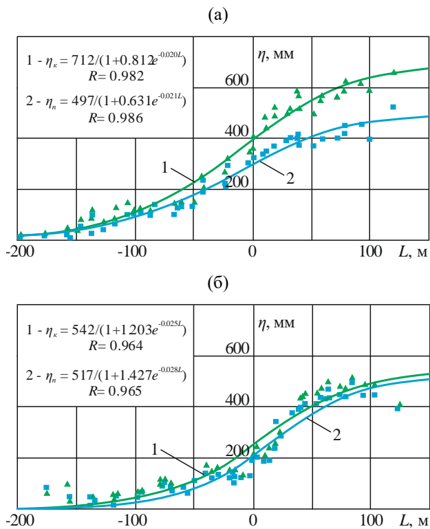
Рисунок 2. Зависимость сдвижения пород ( \eta ) на контуре 159-го (а) и 163-го (б) штреков от расстояния до очистного забоя ( L ) при отработке 157-й и 161-й лав шахтой “Степная”: 1, 2 – усредняющие кривые при сдвижении пород соответственно кровли и почвы; \blacktriangle , \blacksquare – экспериментальные данные; R – корреляционное отношение
