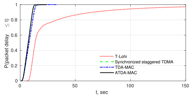
(d) Scenario 4: 20 nodes, 9.2 kb/s channel, 4096 bit packet length
