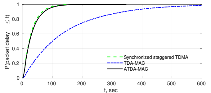
(d) Scenario 4: 20 nodes, 9.2 kb/s channel, 4096 bit packet length
