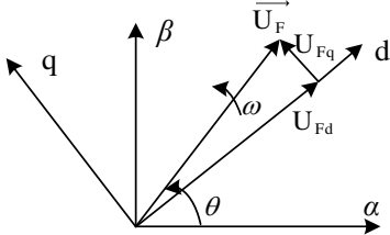
Fig. 4 Voltage vector in dq reference frame
