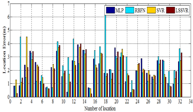
Fig. 12. Model localisation errors
