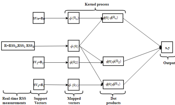
Fig. 5. SVR PD Localisation model
