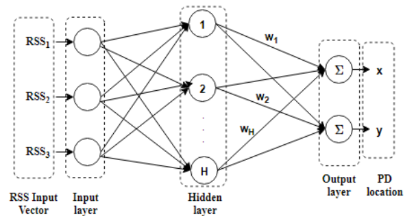
Fig. 4. RBFN PD localisation model
