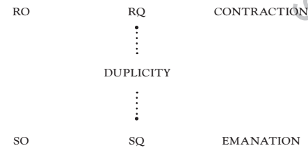
fig IV: tiga radiasi
