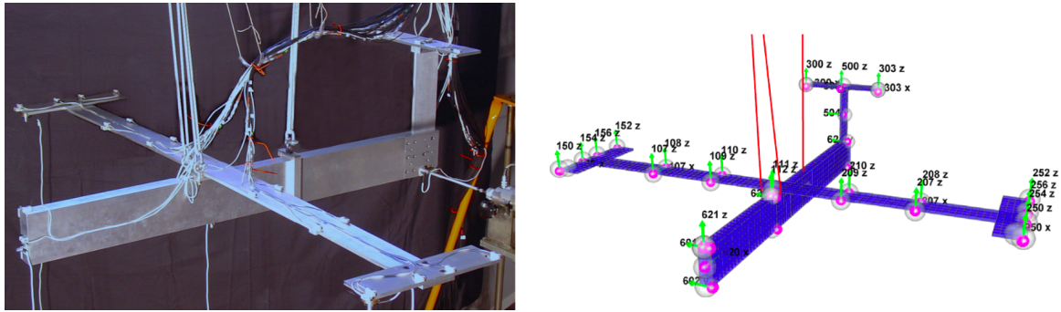
Fig. 1. DLR-AIRMOD structure [15].
