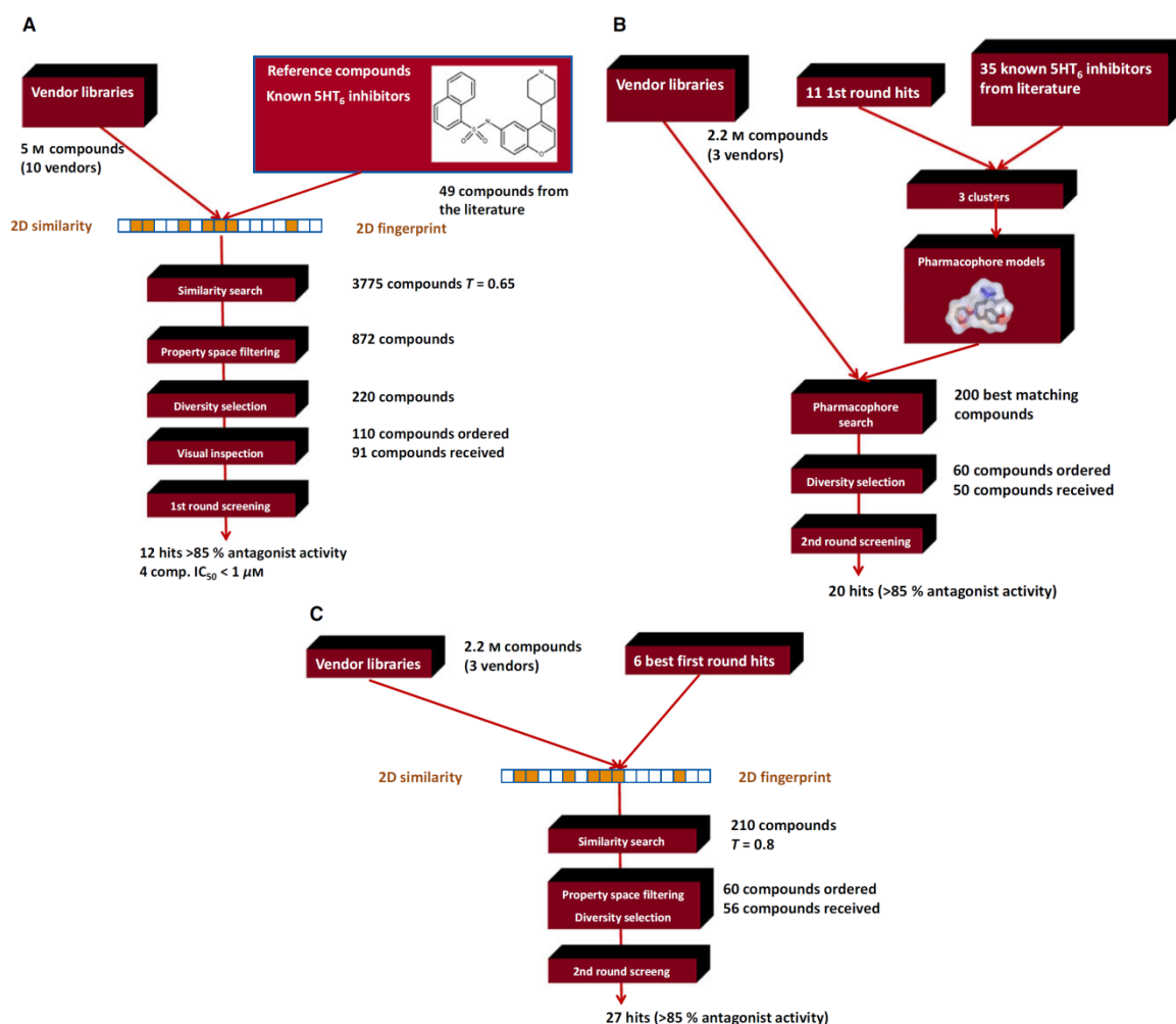
6.ábra Többlépcsős in silico/in vitro szűrési kaszkád az 5-HT 6 fókuszált könyvtár szelektálására és validálására, két szelektációs körben, hasonlósági és farmakofór szűréssel
