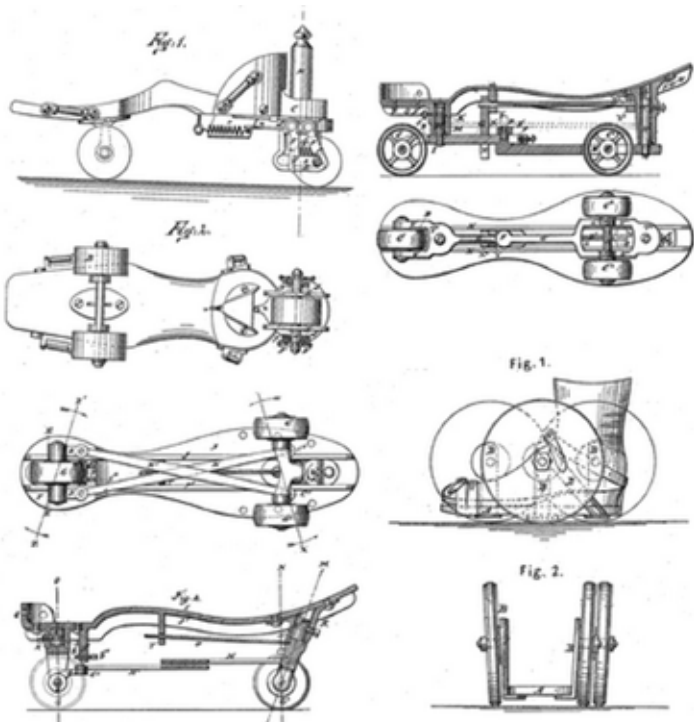
12. ábra Háromkerékű görkorcsolya tervek. A rajzok USA-ban bejegyzett szabadalmi számai: 98117 (1869 év), 177566 (1876), 177 568 (1876), 196230 (1877). (Mitskevichus, Роликовые коньки - roller skates (окончание), 2011)
