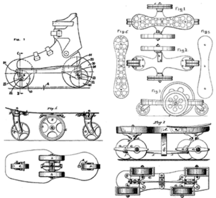
13. ábra Alternatív négykerékű görkorcsolya tervek. A rajzok az USA-ban bejegyzett szabadalmi számai: 188.351 (1877), 233 845 (1880), 280236 (1883) 7758054 (2010)
