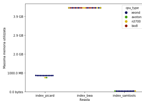
Figura 3.7: Memoria impiegata dalle regole indipendenti dai subsets.
