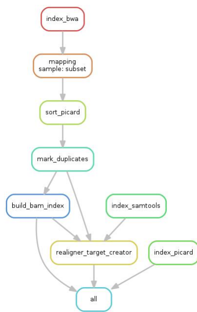
Figura 2.1: Schematizzazione del procedimento implementato nella pipeline.
