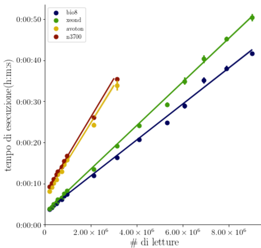
Figura 3.2: Tempi per Build BAM.
