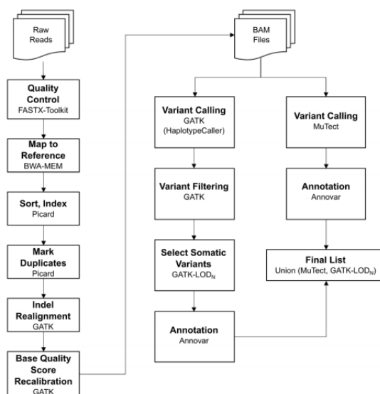
Figura 1.1: Pipeline di GATK-LOD n (presa da [3]).
