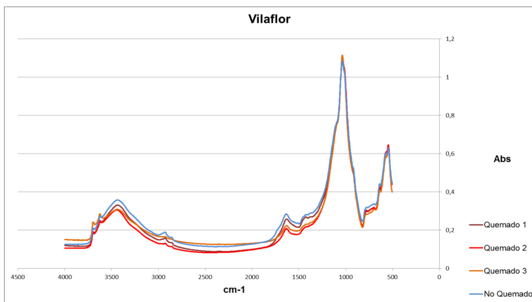
Figura 6. Espectro de FTIR en pastilla de KBr de las muestras Quemado (Q1, Q2 y Q3) y No Quemado (NQ) de Vilaflor (Tenerife), medido en el intervalo espectral entre 4000-500 \text{cm}^{-1} .
