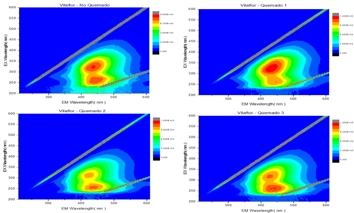
Figura 11. Espectro de fluorescencia de las muestras Quemado (Q1, Q2 y Q3) y No Quemado (NQ) de Vilaflor, medido en un intervalo de excitación entre 200 y 600 nm y un intervalo de emisión entre 210 y 610 nm.
