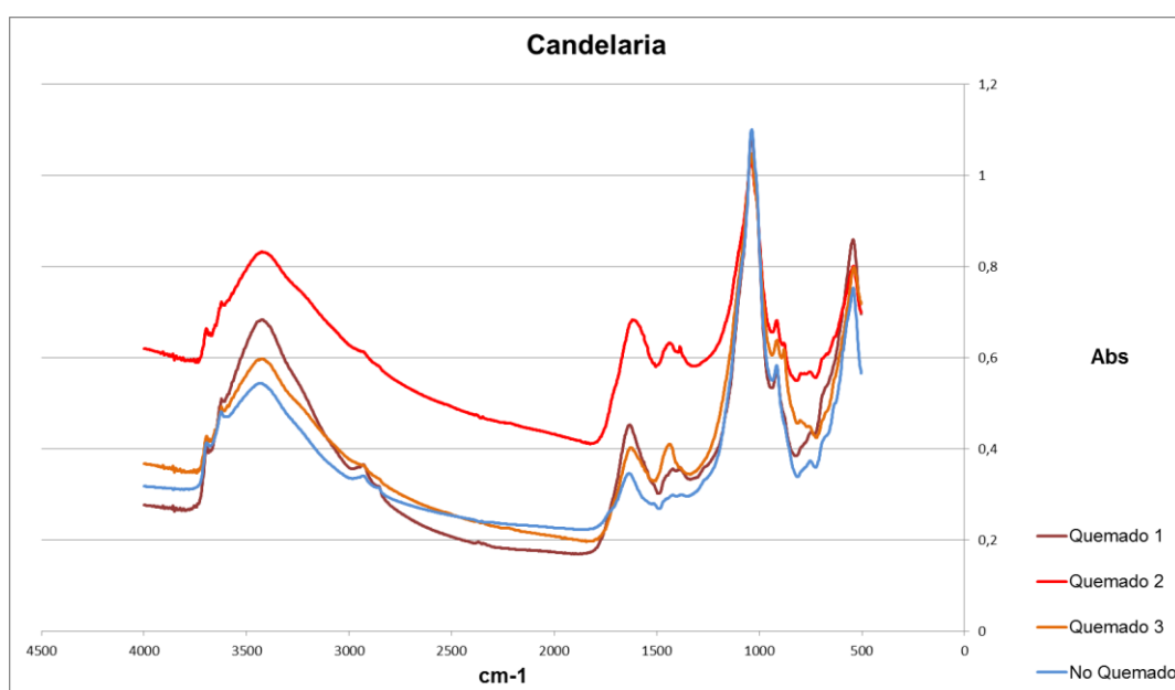
Figura 5. Espectro de FTIR en pastilla de KBr de las muestras Quemado (Q1, Q2 y Q3) y No Quemado (NQ) de Candelaria (Tenerife), medido en el intervalo espectral entre 4000\text{-}500\text{ cm}^{-1} .
