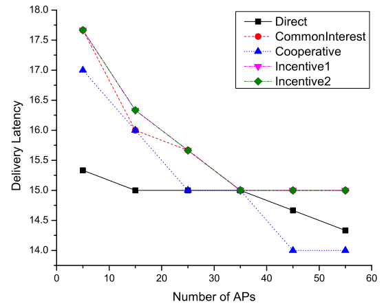
(d) MOBICOM06
