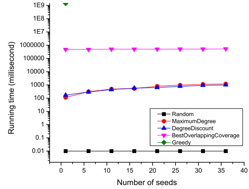
(d) Amazon0302
