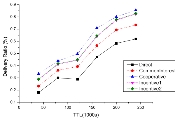
(c) SIGCOMM09
