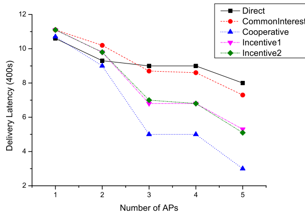
(a) UmassDisel06
