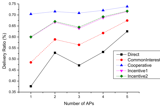
(c) SIGCOMM09
