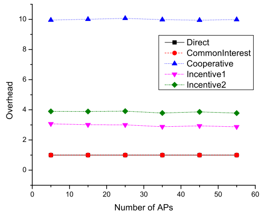
(d) MOBICOM06
