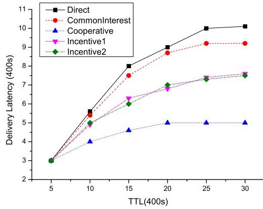
(a) UmassDisel06
