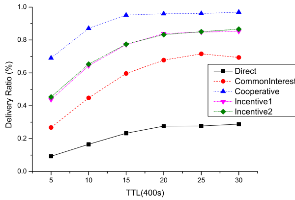
(a) UmassDisel06
