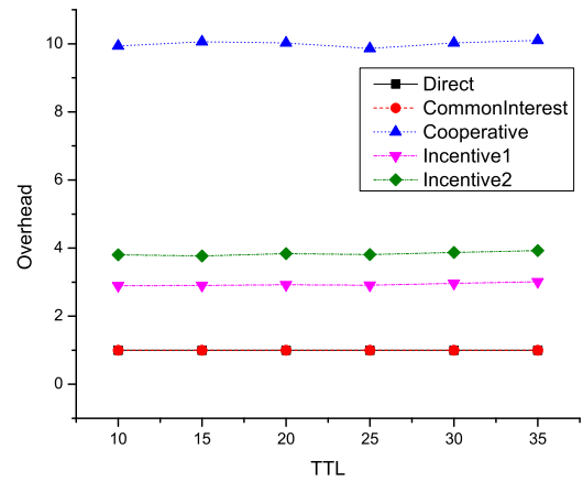
(d) MOBICOM06
