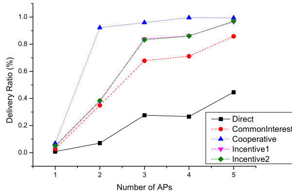
(a) UmassDisel06
