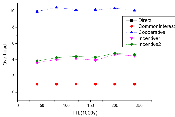
(c) SIGCOMM09
