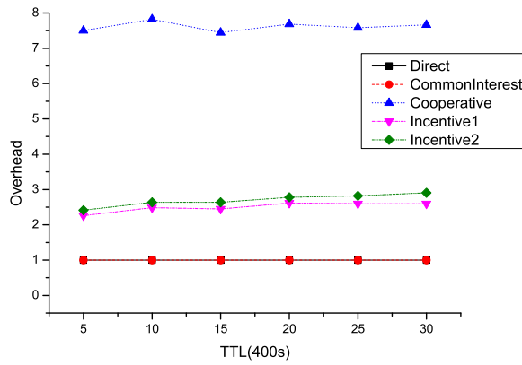
(a) UmassDisel06
