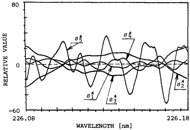
(b) adjoint spectra
