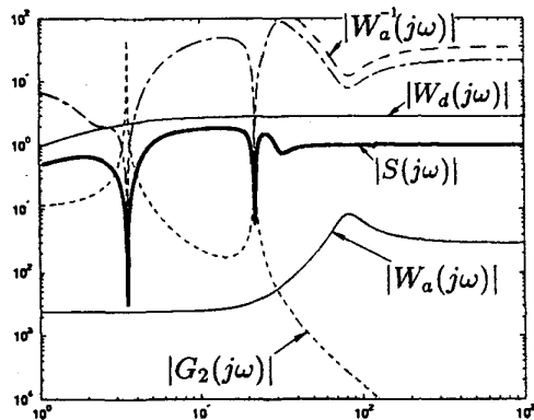
Figure 2: Design result of controller ( |S(j\omega)| , |G_2(j\omega)| , |W_d(j\omega)| , |W_a(j\omega)| )
