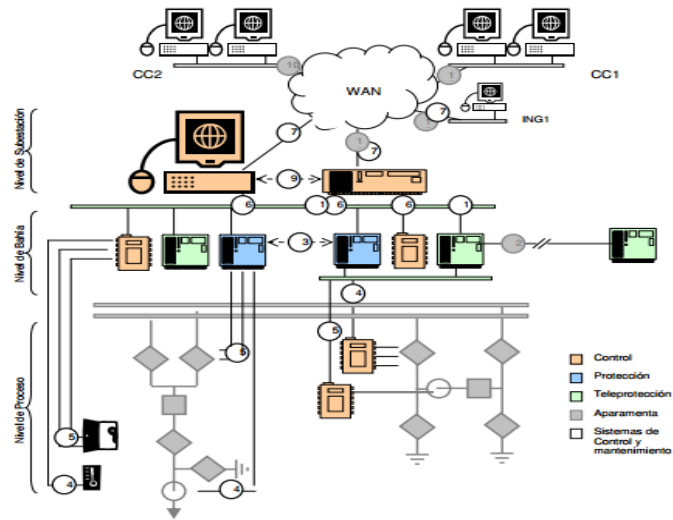
Figura 2 arquitectura genérica de una S/E
