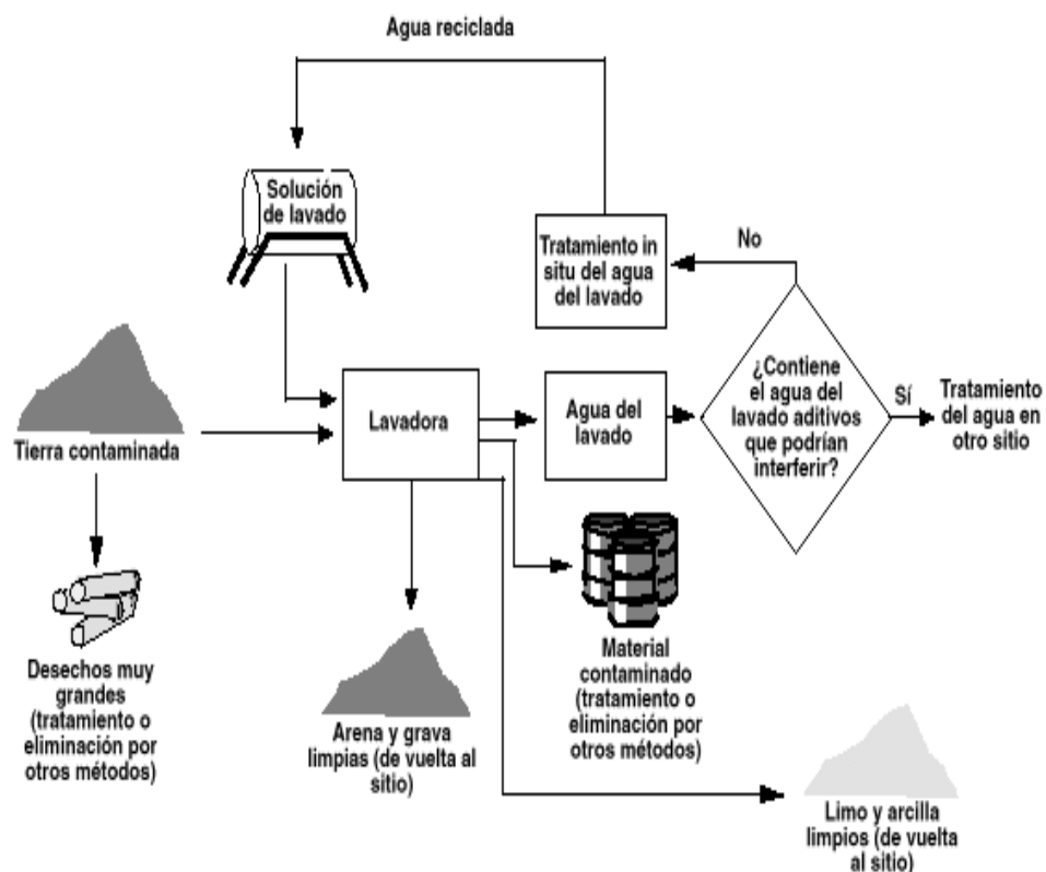
Figura 2.5.- Proceso de extracción con solventes (EPA, 1996)
