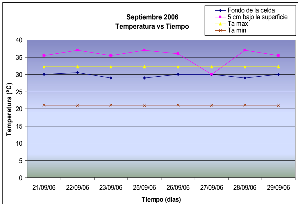
Grafico 5.1.- Temperatura vs. Tiempo, correspondiente al mes de septiembre 2006
