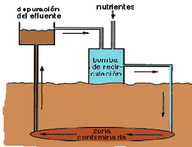
Figura 2.9.- Tratamiento microbiológico in situ (X. Domenech, 1995)
