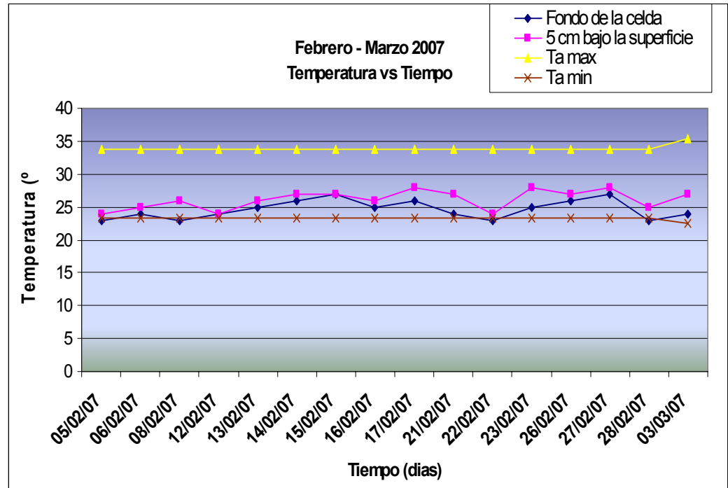
Grafico 5.6.- Temperatura vs. Tiempo, correspondiente al mes de febrero – marzo 2007
