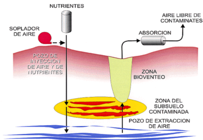
Figura 3.1.- Proceso de Bioremediación in situ de agua y suelo (Evaluación de Riesgos y Restauración Ambiental, 2001).
