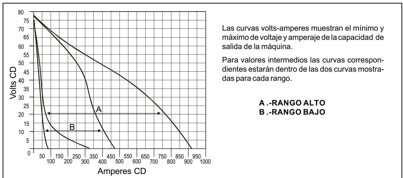
FIGURA 2-1 CURVAS VOLTS-AMPERES.
