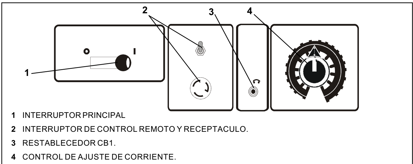
FIGURA 4-1 CONTROLES
