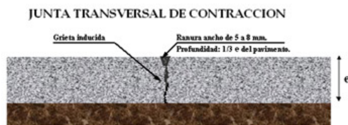
Figura 23. Junta de Contracción.
