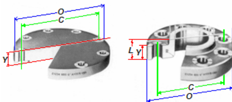
FIGURA 3.5. BRIDA CIEGA Y BRIDA DESLIZANTE
