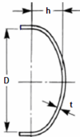
FIGURA 3.4. CARA LATERAL ELIPSOIDAL
