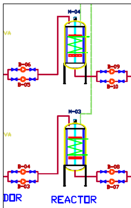
FIGURA 2.15. DISEÑO DEL PROCESO DE REACCIÓN
