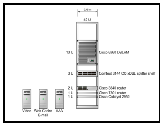
Figura 3. Ubicación equipos ADSL en CO
