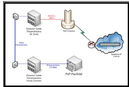
Figura 4. Diagrama enlace a Internet
