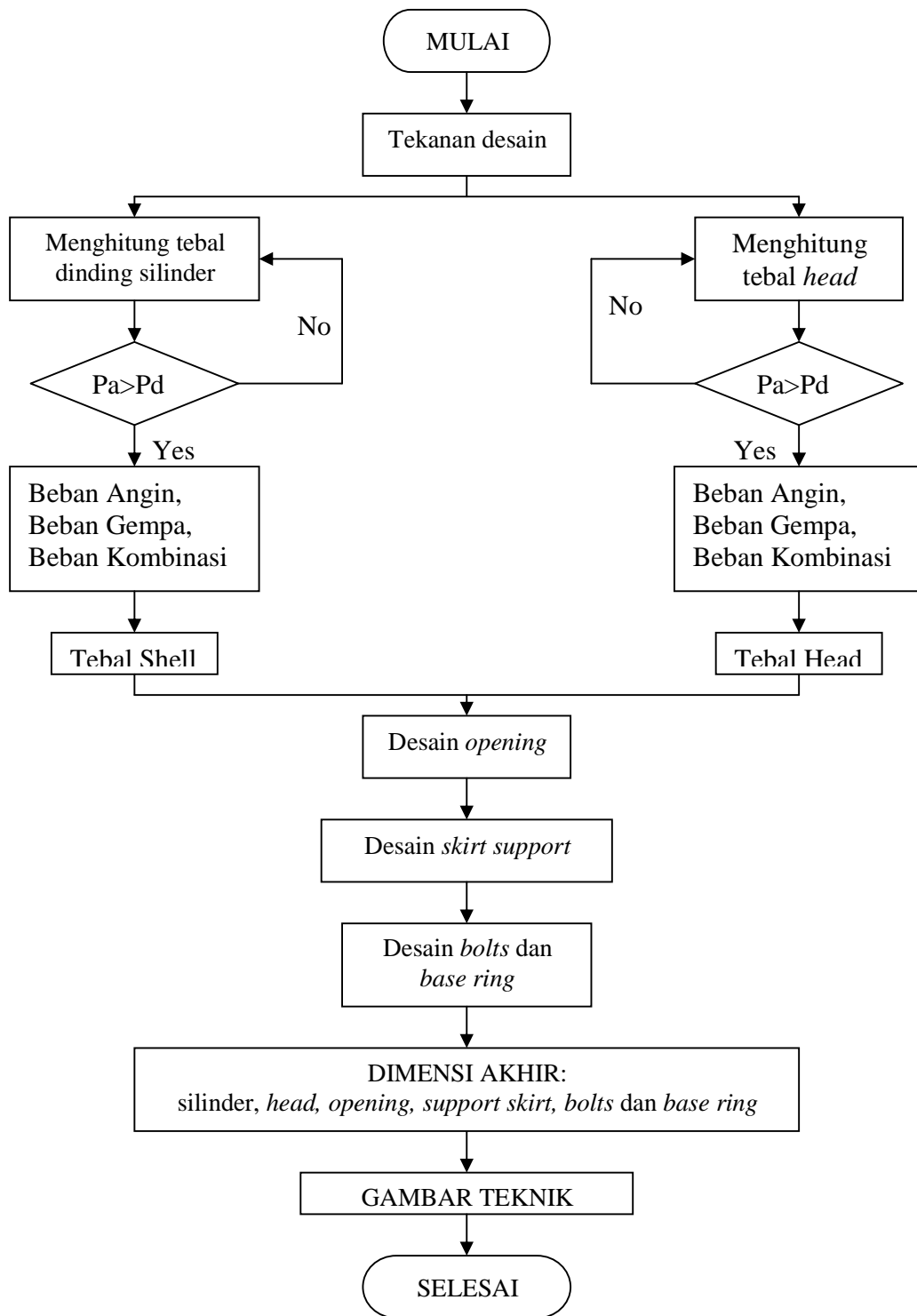
Gambar 3.8 Alur Perancangan
