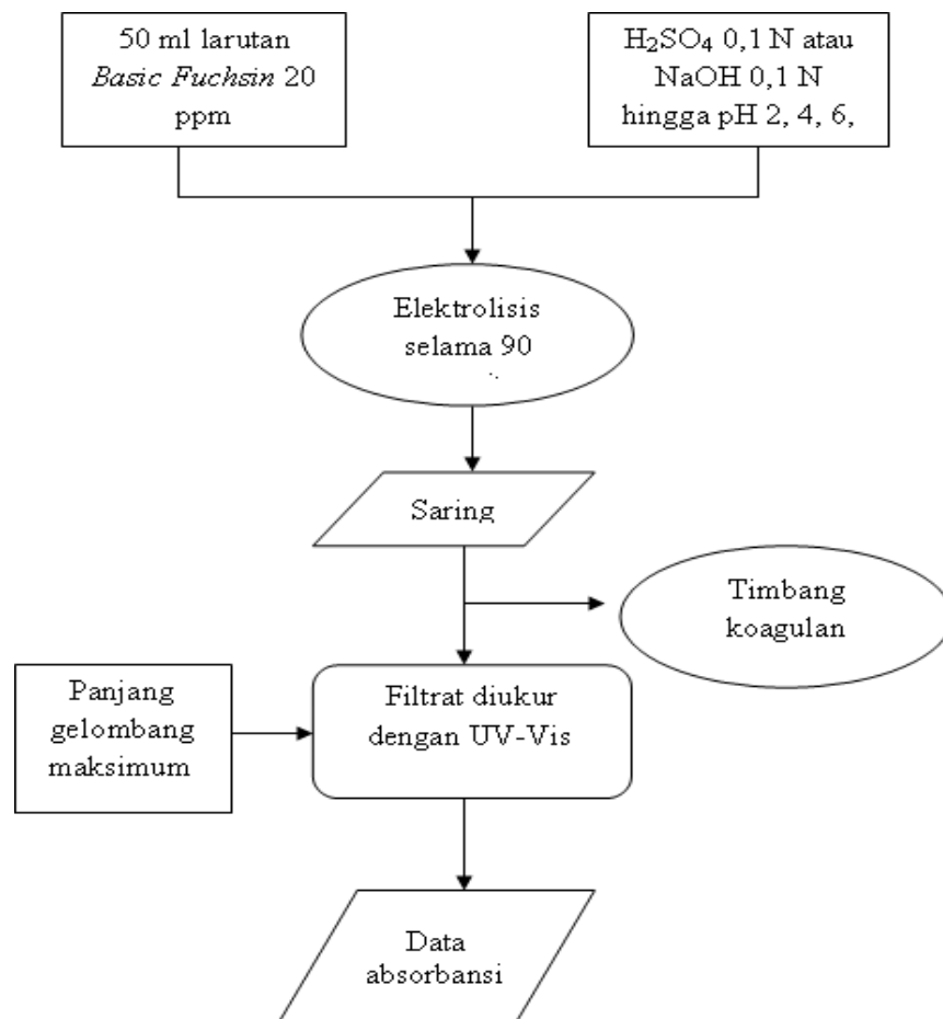
Gambar 2. Skema kerja elektrokolorisasi dalam penentuan pH optimum larutan sampel Basic Fuchsin .
