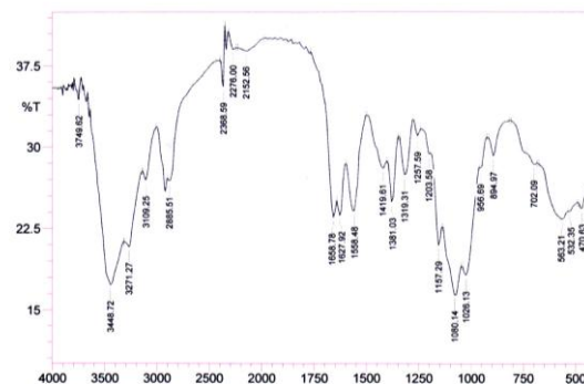
Gambar 1. Spektra FTIR pada produk Khitosan
