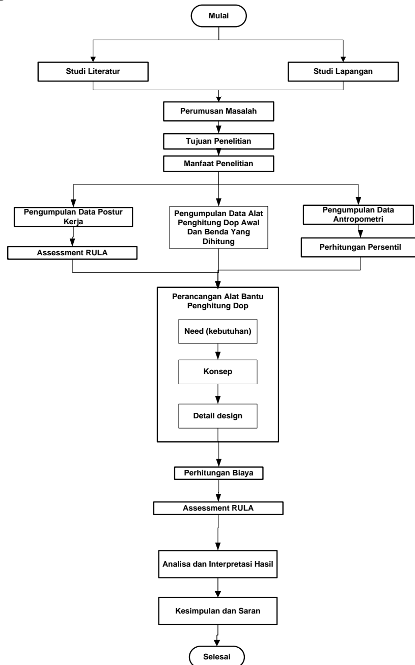
Gambar 1. Metodologi penelitian
