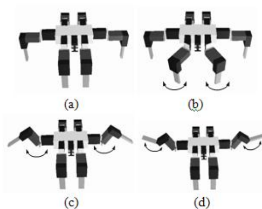
Gambar 6. Pergerakan servo dalam robot: (a) posisi robot mula-mula; (b) pergerakan hip servo ; (c) pergerakan knee servo ; (d) pergerakan ankle servo
