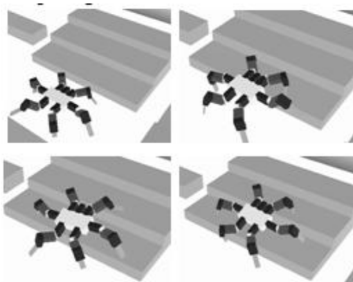
Gambar 22. Simulasi robot menaiki tangga dengan tinggi 8 cm dan lebar 25 cm
