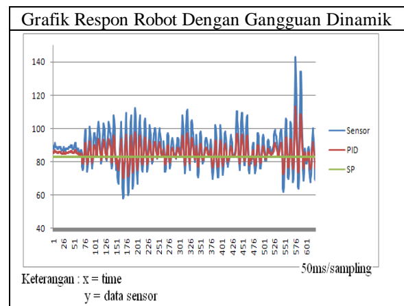
Gambar 19. Respon Robot Titik Tumpu Bawah
