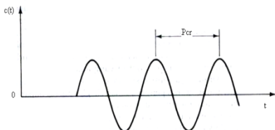
Gambar 3. Kurva Tuning PID Ziegler Nichols orde 2.
