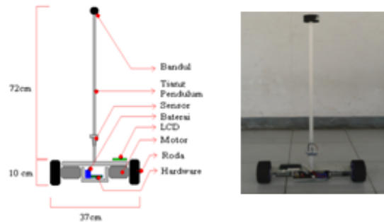
Gambar 5. Desain Mekanik
