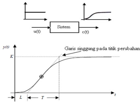
Gambar 2. Kurva Tuning PID Ziegler Nichols orde 1.
