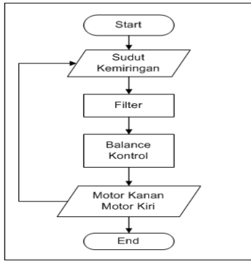
Gambar 7. Cara Kerja Robot
