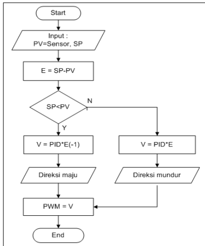
Gambar 8. Direksi Gerakan Robot
