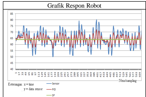
Gambar 17. Respon robot titik tumpu atas
