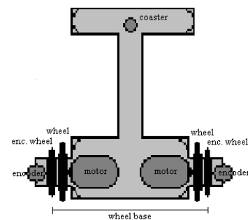
Gambar 1. Desain robot
