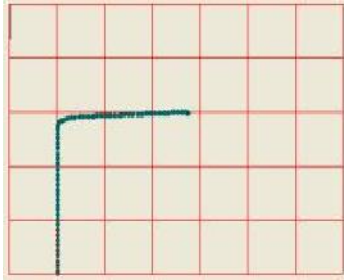
Gambar 9. Jalur berdasarkan perhitungan odometry dari robot pada path ketiga
