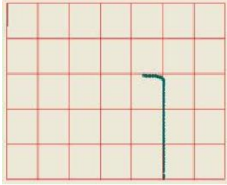
Gambar 23. Jalur berdasarkan perhitungan odometry dari robot pada path kedua
