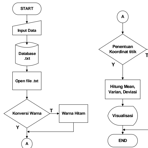
Gambar 3.3 Flowchart Visualisasi
